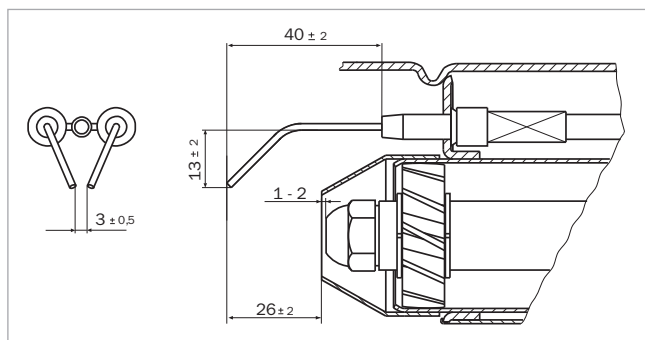
Abb. 70: Zündelektroden prüfen
