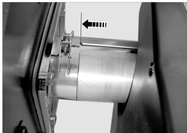
Abb. 11: Brenner bis zum Anschlag einschieben
