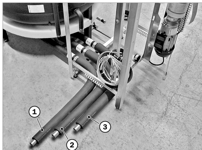
Abb. 19: Heizungsanschlüsse montieren
