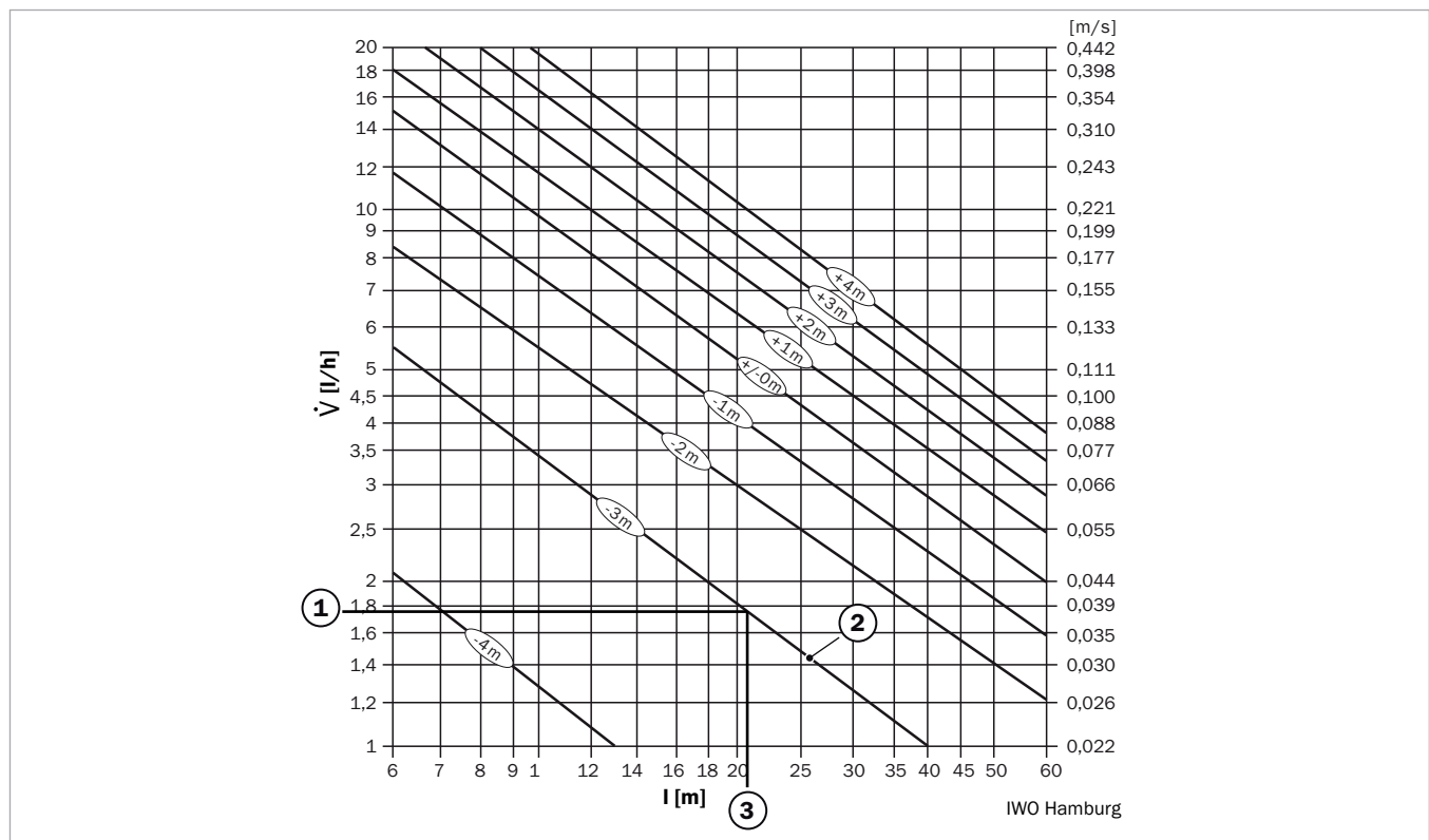
Abb. 38: Maximale Leitungslänge im Einstrangsystem in Abhängigkeit von der Förderhöhe
