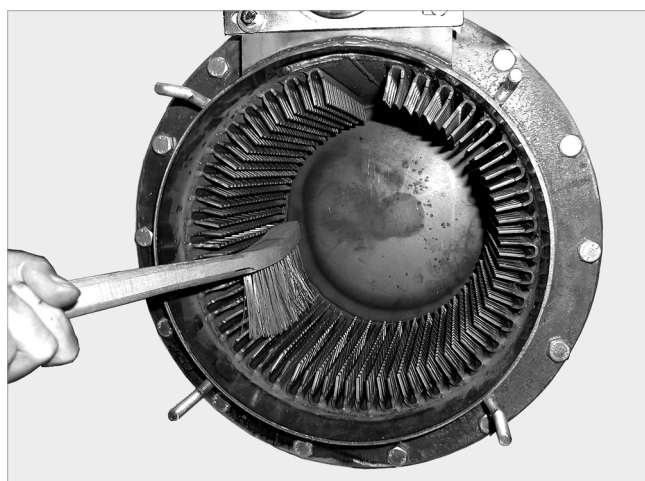
Abb. 71: Abgas-Wärmetauscher reinigen
