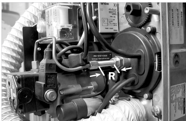
Abb. 56: Rezirkulationsspalt einstellen
