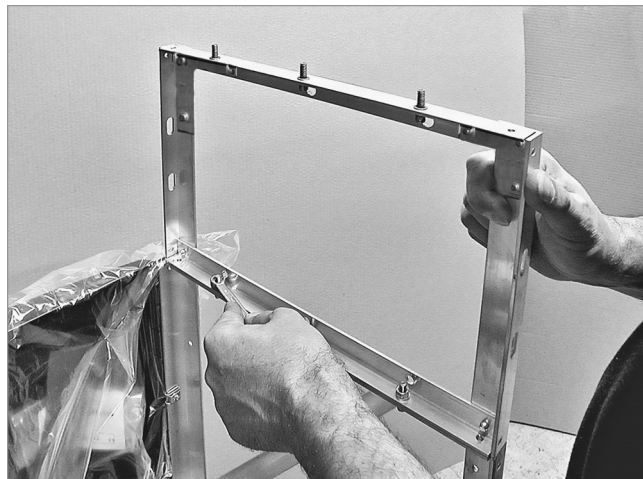
Abb. 15: Konsolenaufsatz montieren
