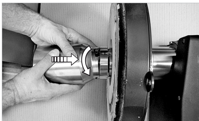
Abb. 13: Flammrohr befestigen
