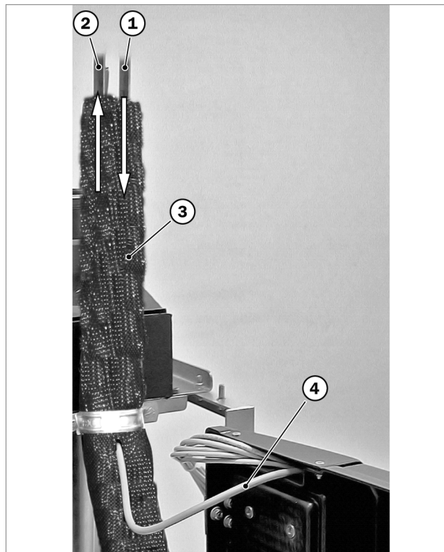
Abb. 36: Schnellmontagerohr anschließen
