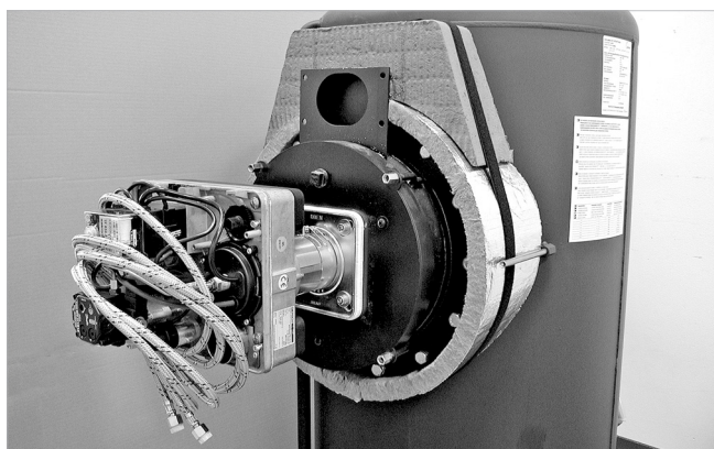
Abb. 14: Montage Brennraumbür
