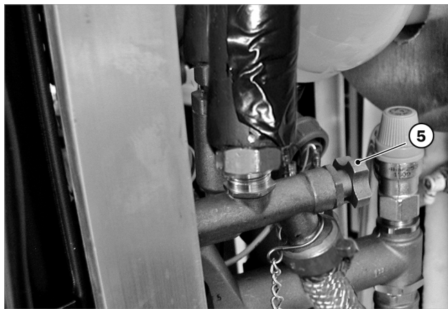
Abb. 61: Spülhahn am Solar-Vorlauf
