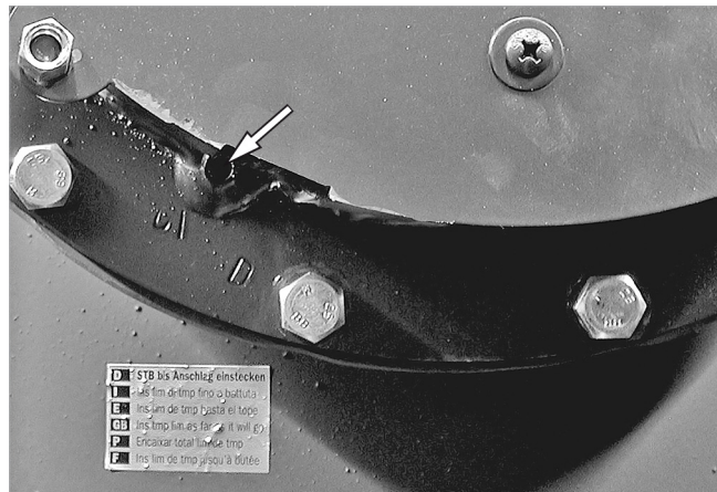
Abb. 31: mSTB einstecken
