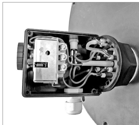
Netzkabel anschließen
