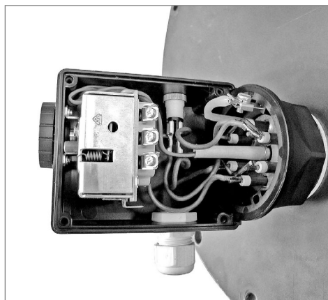
Voedingskabels aansluiten
