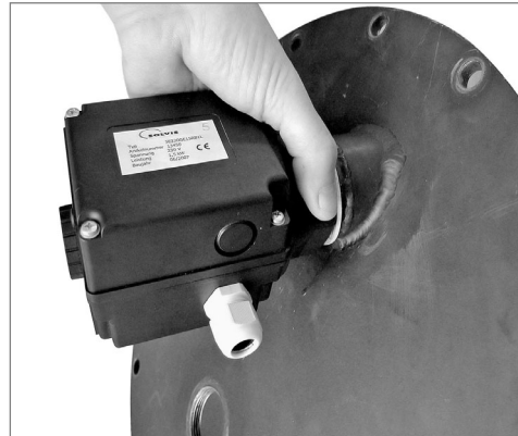
E-Heizstäbe einschrauben
