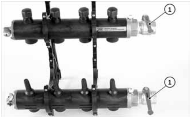
Abb. 8: Absperrhähne schließen
