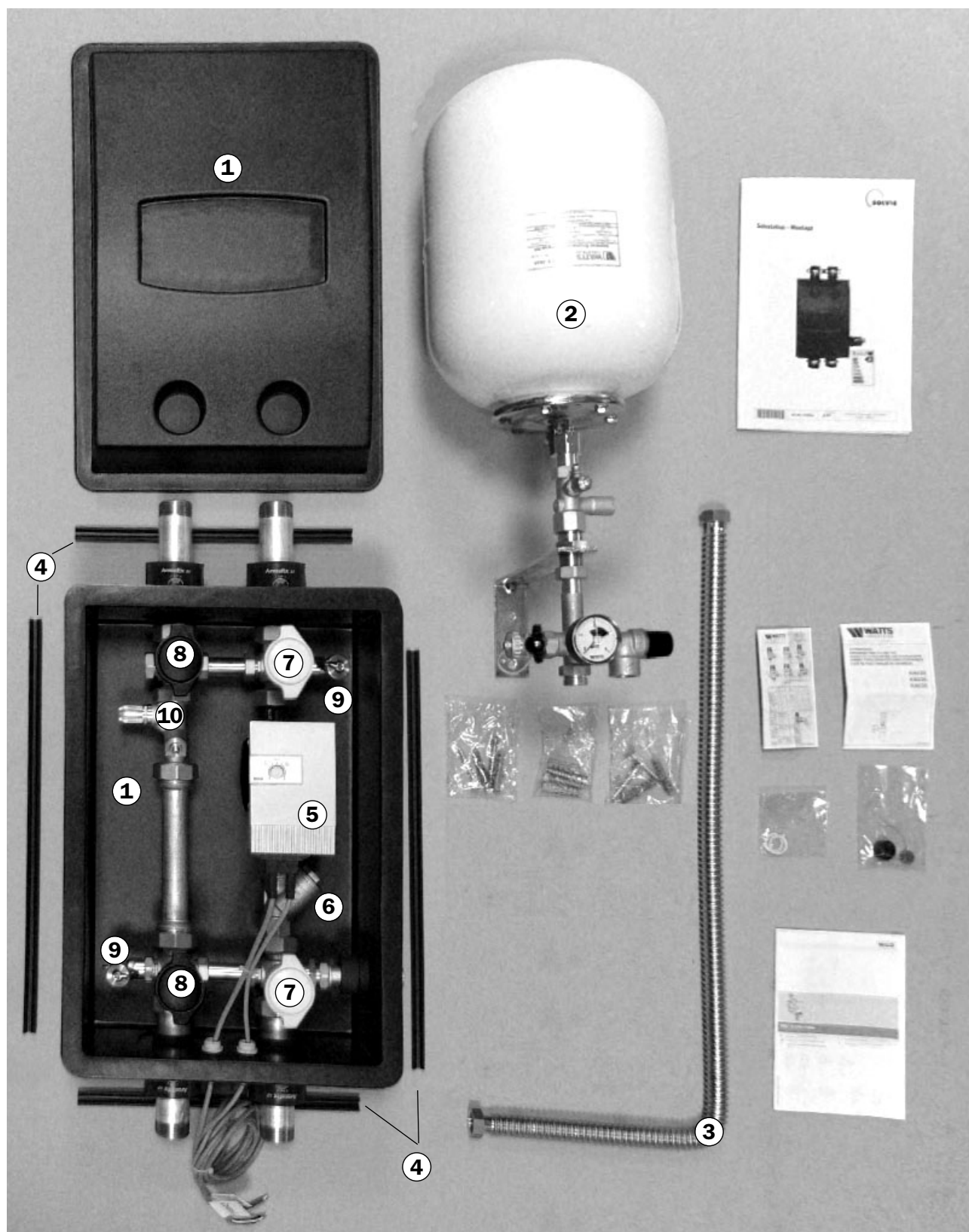
Lieferumfang Solestation
