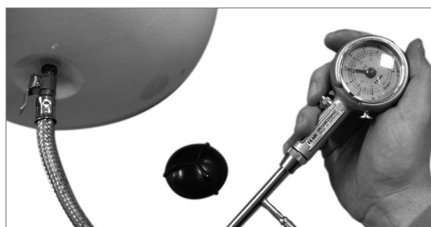
Sole-Ausdehnungsgefäß
