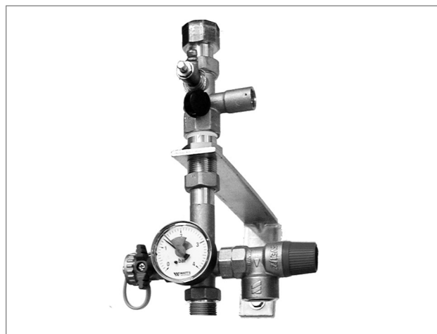
Sicherheitsgruppe montiert
