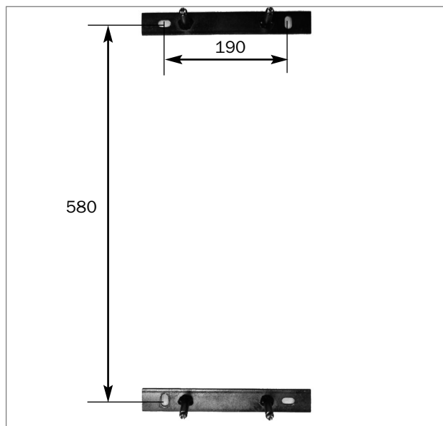
Wandhalter montieren
