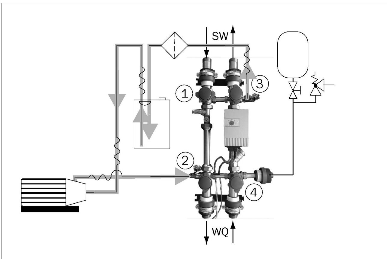
Wärmequelle spülen
