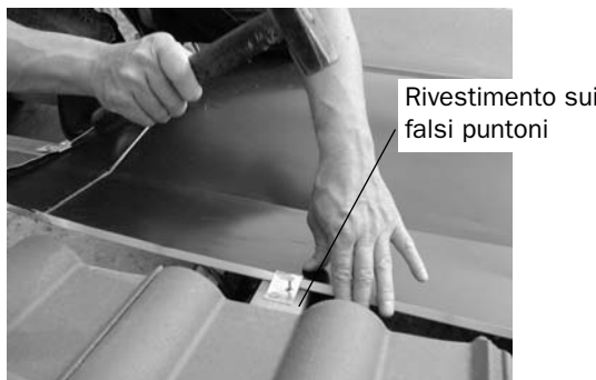
Fig. 118: Fissare la lamiera superiore sul lato superiore del collettore
