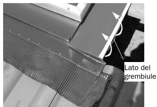
Fig. 21: Piegarlo il lato del grembiule sopra quello della lamiera laterale
