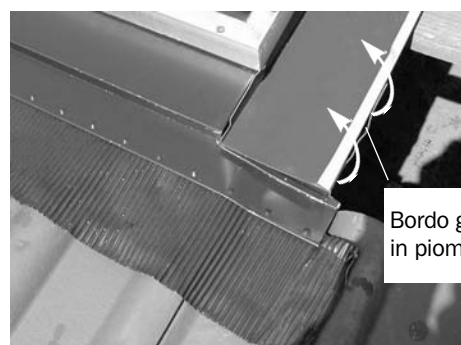
Fig. 60: Piegar il bordo del grembiule su quello della lamiera laterale
