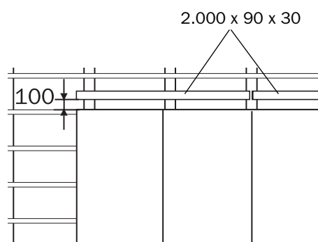
Fig. 61: Montare i pannelli in legno
