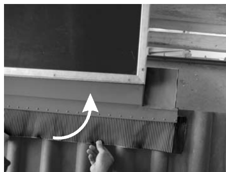
Fig. 12: Inserire il grembiule a destra con l'angolo
