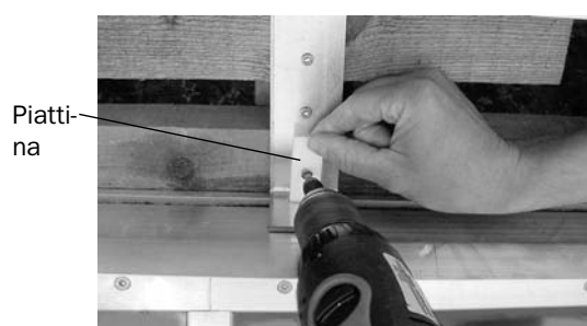
Fig. 135: Fissaggio superiore del collettore
