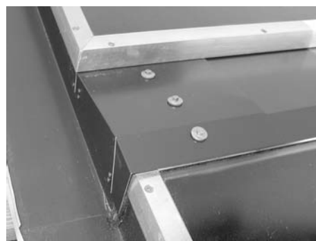
Fig. 175: Lamiera intermedia di sinistra montata
