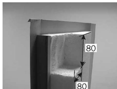
Fig. 66: Solo per due collettori integrali: tagliare l'angolo sul lato dei collegamenti
