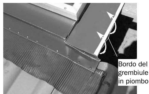
Fig. 98: Piegare il bordo del grembiule su quello della lamiera laterale
