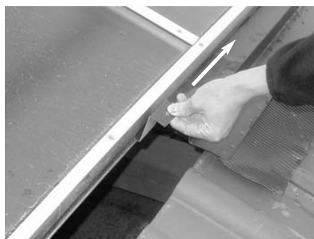
Fig. 13: Inserire due fissaggi per grembiule
