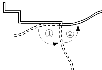
Fig. 11: Ruotare il grembiule in piombo
