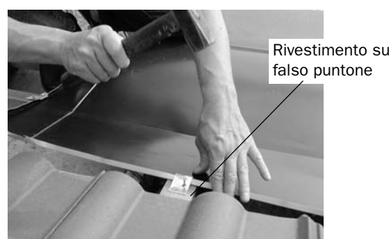
Fig. 30: Fissare la lamiera superiore sul lato superiore del collettore
