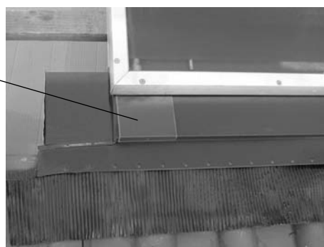
Fig. 16: Grembiule di sinistra con angolo
