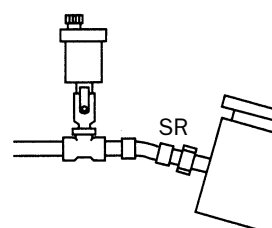
Fig. 212: Collegamento superiore con sfiatatoio rapido
