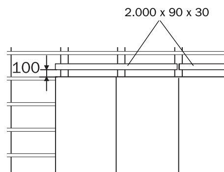
Fig. 22: Montare i pannelli in legno
