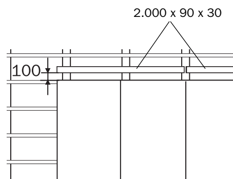
Fig. 110: Montare i pannelli in legno
