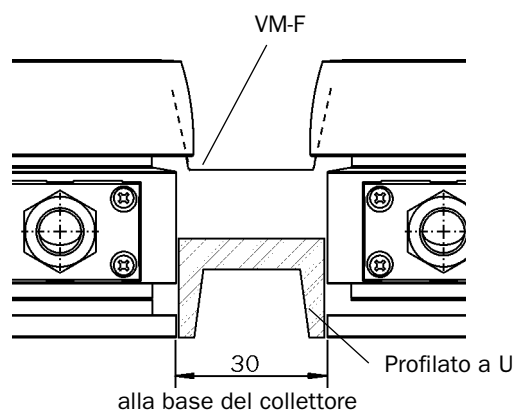
Fig. 131: Sezione B-C (dalla figura 125)
