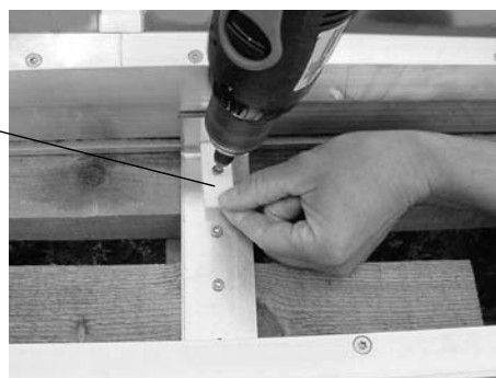
Fig. 86: Fissaggio inferiore del collettore
