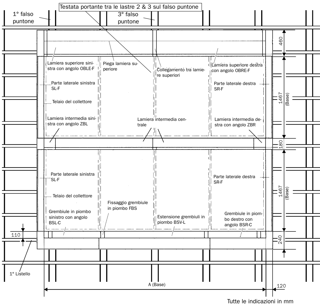
Fig. 77: Misure dell'impianto (qui come esempio: 2 x F 552)
