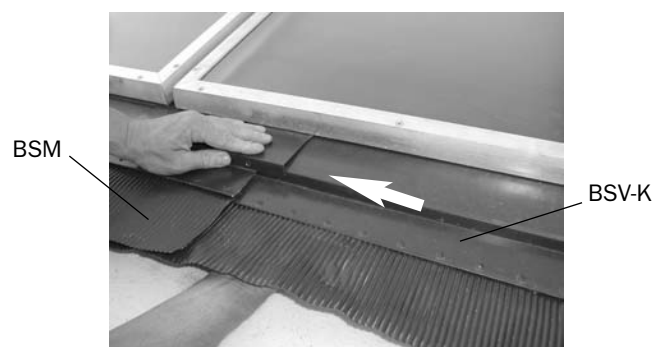
Fig. 51: Spingere il grembiule 4
