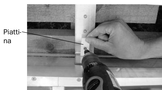
Fig. 135: Fissaggio superiore del collettore
