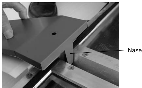
Fig. 68: Posizionare la connessione con l'aletta per la lamiera superiore, allineare ed avvitare con forza il tutto
