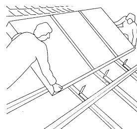
Fig. 128: Inserire il collettore inferiore
