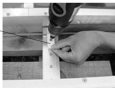
Fig. 137: Fissaggio inferiore del collettore
