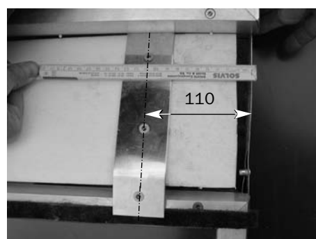
Fig. 103: Inserire la parte inferiore dell'angolo della lamiera intermedia
