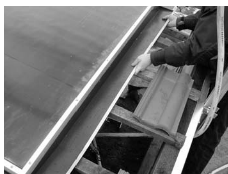
Fig. 59: Inserire le lamiere laterali e posizionarle sull'angolo del grembiule
