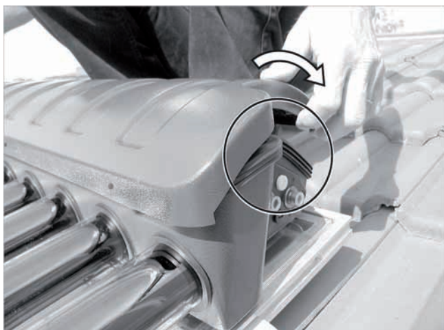
Abb. 1: Gehäusedeckel von schräg oben einsetzen
