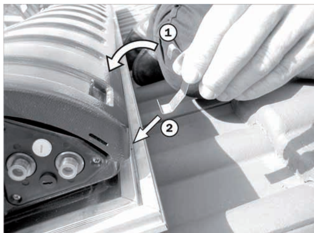
Abb. 3: Klammern einsetzen
