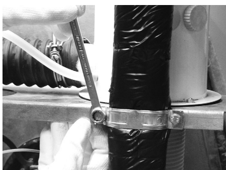
Abrazadera de fijación del conducto solar
