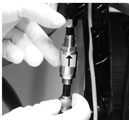
Rückschlagklappe einsetzen
