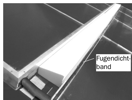
Kollektoren mit Zwischenblechstützen und Fugendichtband
