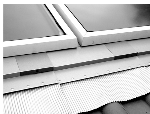
Nächste Bleischürze eingelegt, Fixierungen positioniert
