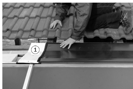
Unterteil des Oberblechverbinders (1) und rechte Oberblechecke einfügen
