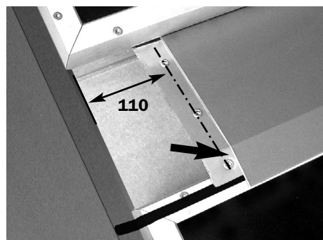
Unterteil Zwischenblechecke in das Zwischenblech eingeschoben
