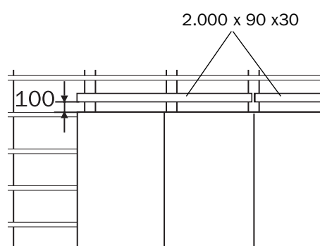
Holzbretter montieren
