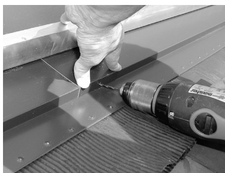
Bleichürzenfixierung andrücken, vorbohren und verschrauben
