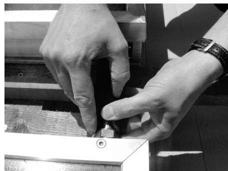
Kollektorverbinder KV-F-Ü am oberen Kollektor verschraubt
