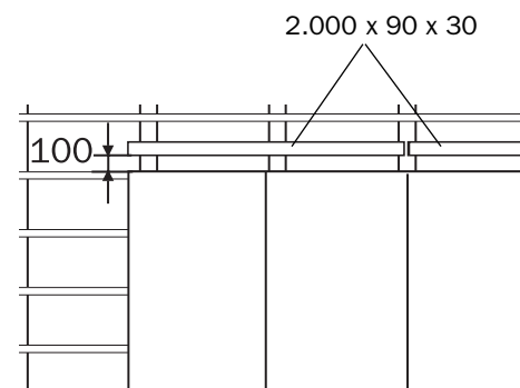
Holzbretter montieren
