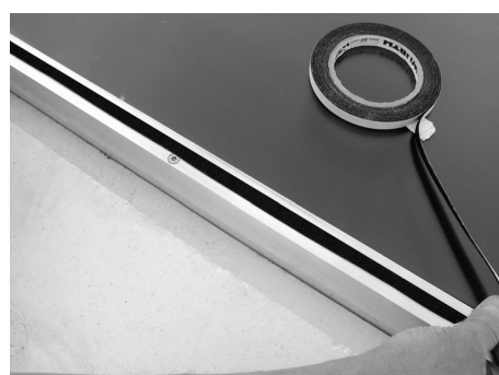
Auf unterem Kollektor Fugendichtband mittig auf dem Profil durchgehend aufkleben
