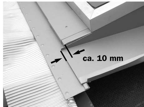
Seitenblech einfügen und über die Bleischürzenecke legen
