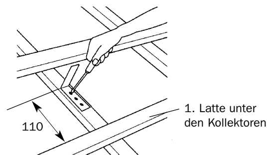
Untere Montagewinkel montieren
