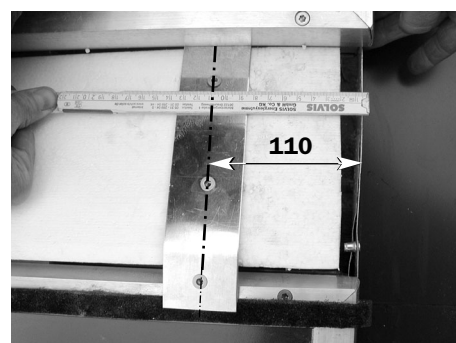
Unterteil Zwischenblechecke einlegen
