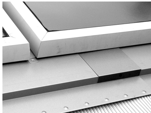
Bleischürzenfixierung zurückgeschoben und positioniert
