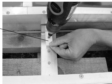
Befestigung des Kollektors unten
