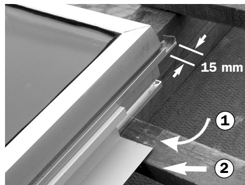
Verbindungsblech einlegen
