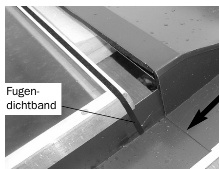
Rechte Oberblechecke in Seitenblech einschieben
