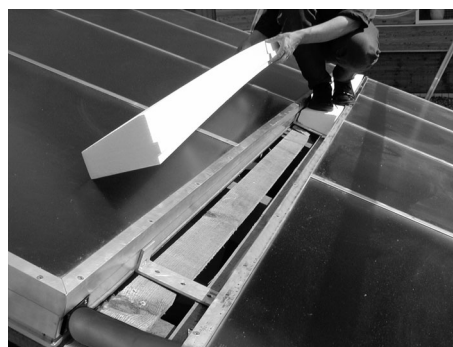
Zwischenblechstützen einlegen
