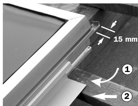
Verbindungsblech einlegen
