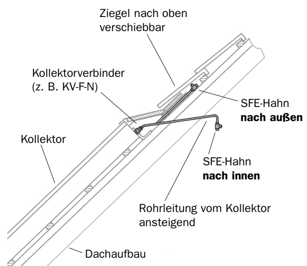
Entlüftung nach innen oder außen geführt
