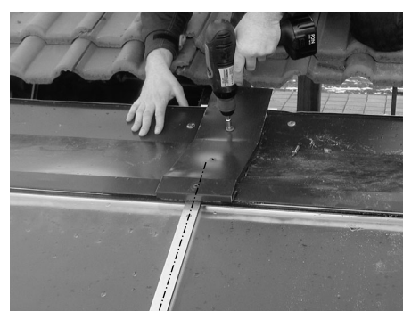
2. Oberblech und Oberblechverbinder auflegen, ausrichten und verschrauben
