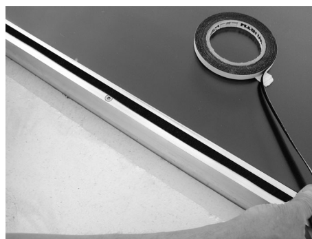
Fugendichtband mittig auf dem Profil durchgehend aufkleben
