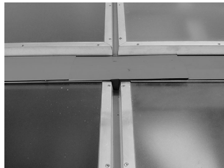
Kreuzstoß fertig montiert
