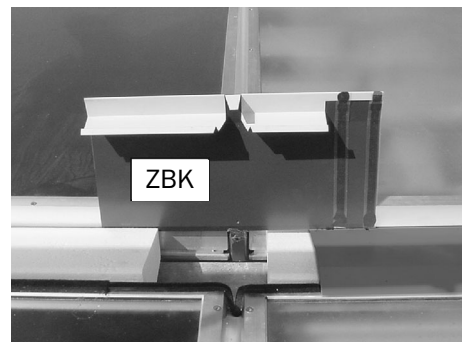
Kreuzungsstück ZBK einlegen
