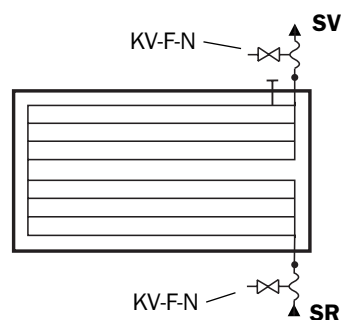
Ein Standardkollektor
