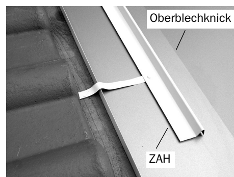
Ziegelanhebung richtig aufgelegt
