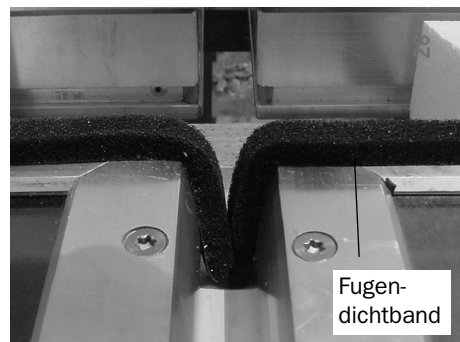
Stoß V-förmig umkleben
