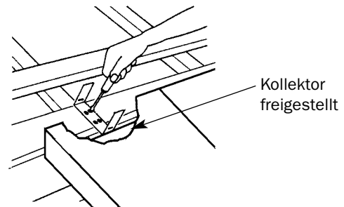
Kollektordistanzstücke setzen
