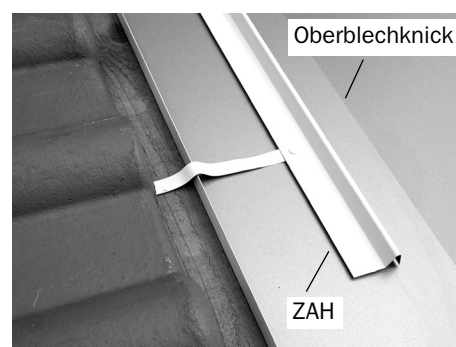
Oberblechknick ZAH Ziegelanhebung richtig aufgelegt
