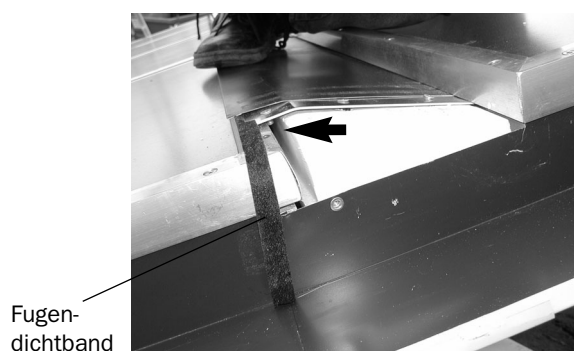
Zwischenblech Mitte eingesetzt
