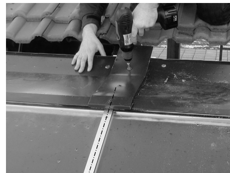
Oberblechverbinder auflegen, ausrichten und verschrauben
