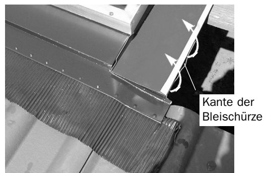
Bleischürzenkante über Seitenblechkante biegen
