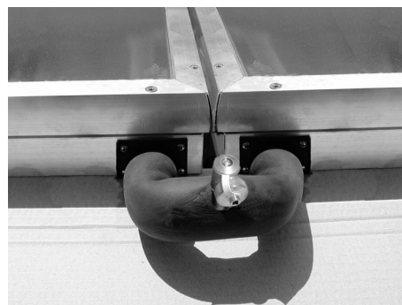
Verbindung Kollektoren nebeneinander
