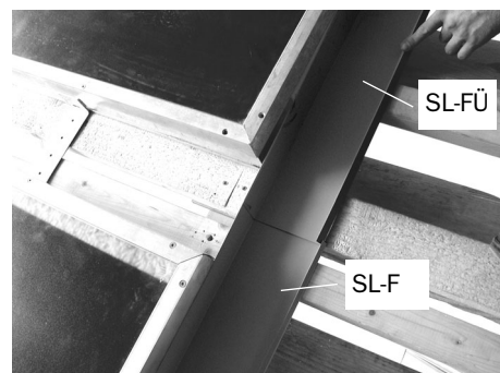
Obere Seitenbleche SL-FÜ montieren
