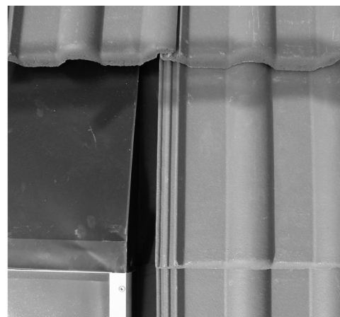
Eindeckung oben und seitlich
