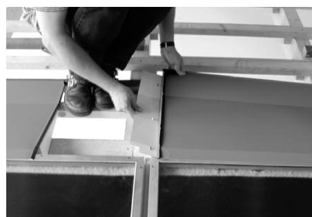
Unterteil vom Oberblechverbinder mit Nase und linkes Oberblech montieren
