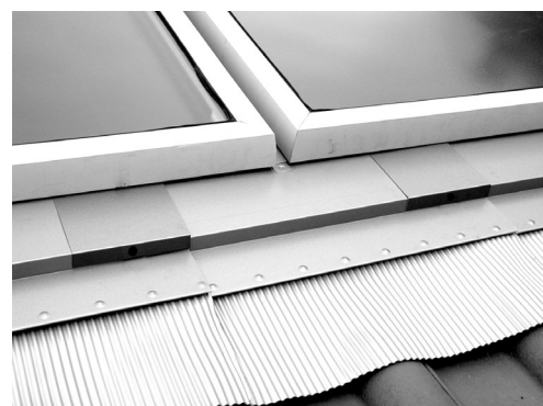
Nächste Bleischürze eingelegt, Fixierungen positioniert
