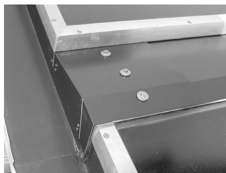
Linke Zwischenblechecke montiert
