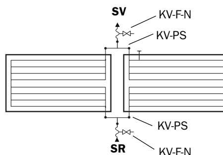
Zwei Standardkollektoren parallel verschaltet
