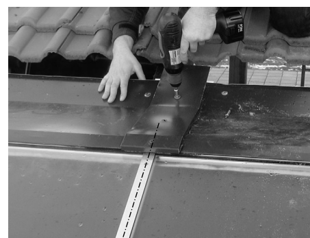
Oberblechverbinder auflegen, ausrichten und verschrauben
