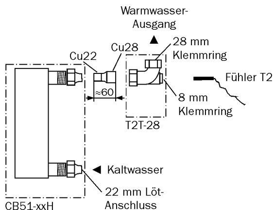
Bild 6: Position des Fühlers T2 mit T-Stück T2T-28
