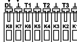
Anschlussplan WES
