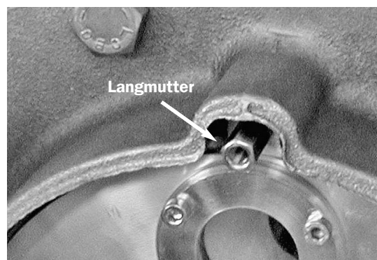
Aufgesetzter Brenner mit Langmutter
