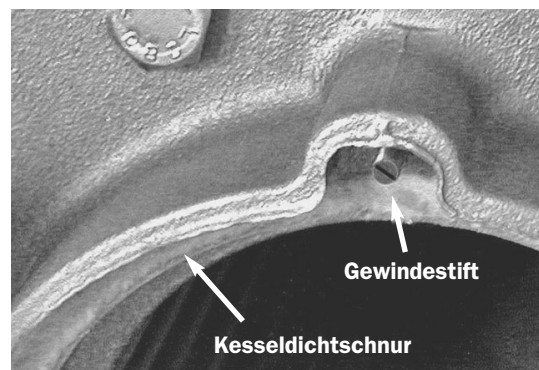
Gewindestift am Flansch
