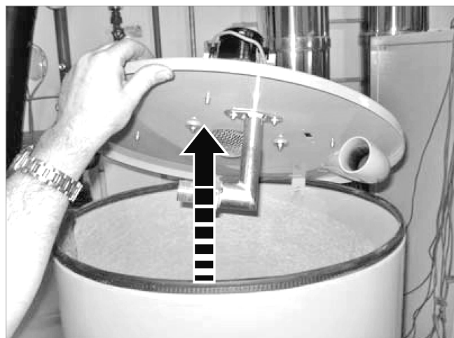
Abb. 1: Alte Saugturbine entfernen
