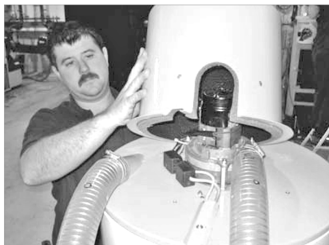
Abb. 10: Haube der Saugturbine aufsetzen
