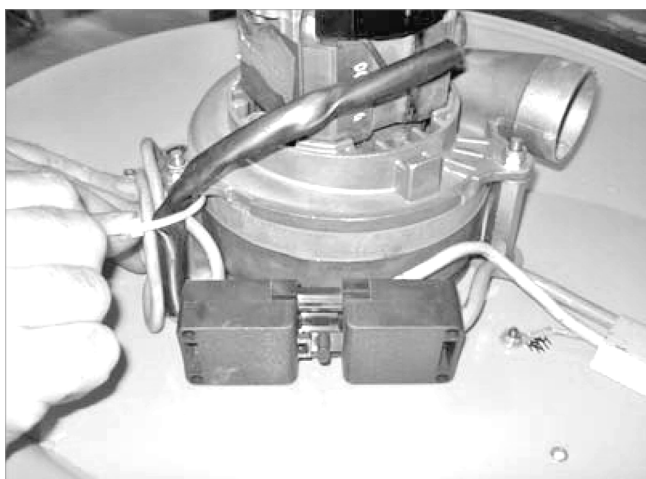
Abb. 7: Kabel fixieren
