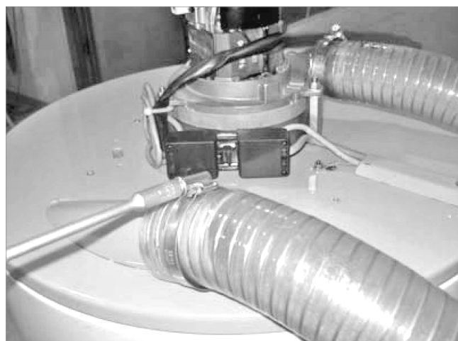
Abb. 9: Pelletschlauch an Behälterdeckel anschließen
