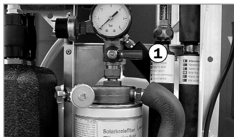
Llave de bola sobre el filtro solar cerrada
