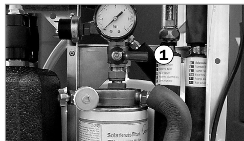
Kugelhahn über dem Solarfilter geschlossen
