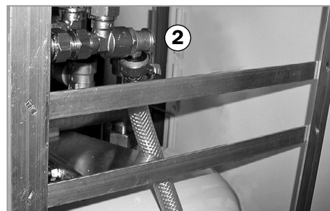
Spölschlauch am Spöhlhahn angeschlossen
