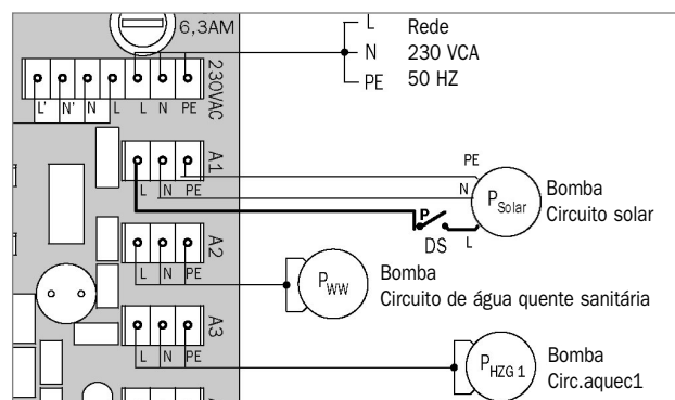
Secção do esquema de ligações: Ligação do pressostato (DS) com a bomba solar
