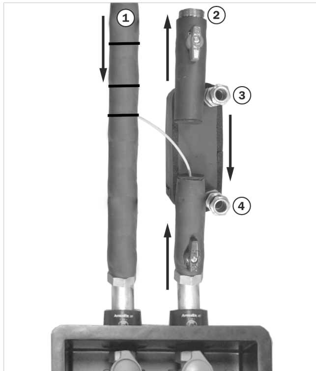
Abb. 3: Plattenwärmeübertrager montiert
