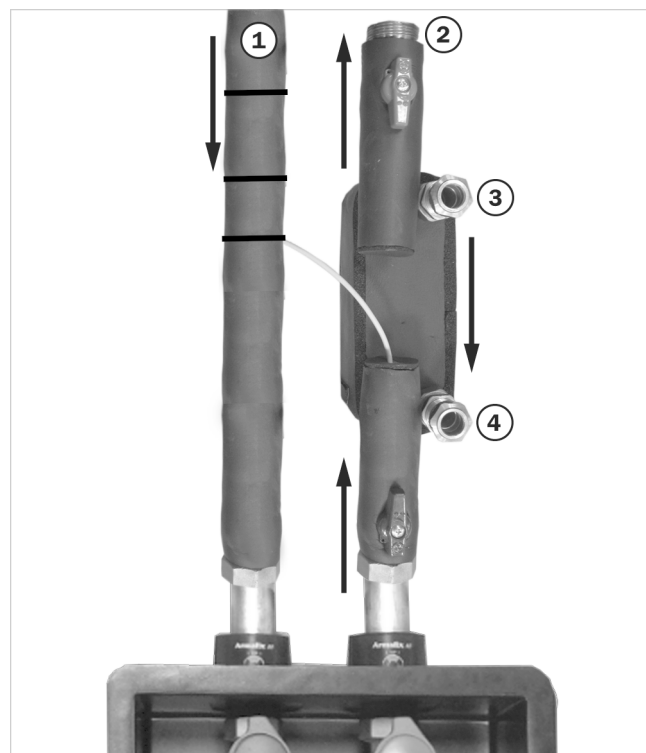
Abb. 5: Plattenwärmeübertrager montiert
