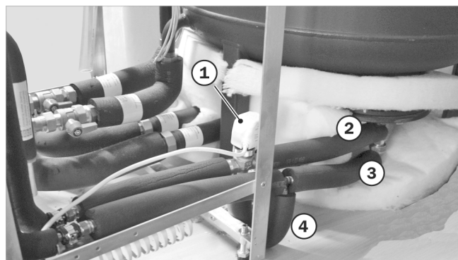
Abb. 7: Dreiwegeumschaltventil montiert
