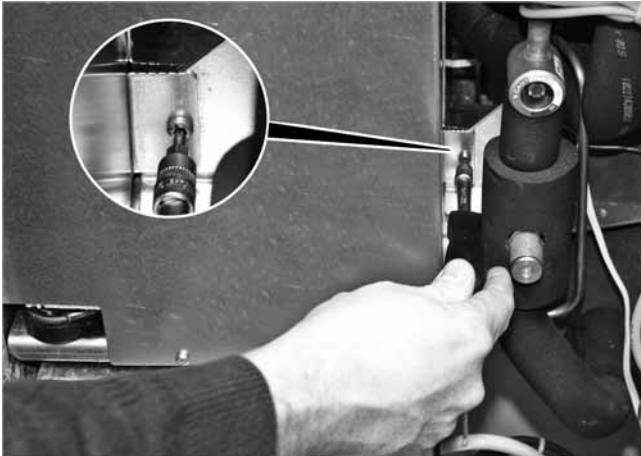
Abb. 7: Am Konsolensteg verschrauben
