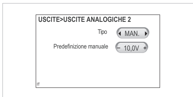
Fig. 16: Impostazione di „Predefinizione manuale“ su 10 V
