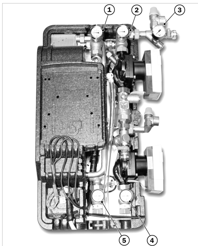
Fig. 1: Valvole di sicurezza montate
