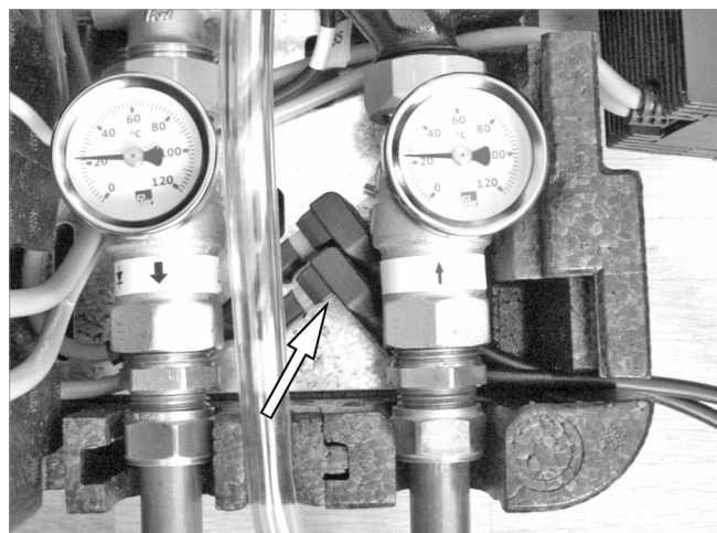
Fig. 5: Collegamento dei connettori Molex
