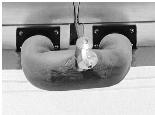
Fig. 10: Esempio su SolvisFera Diagonal con valvola SFE
