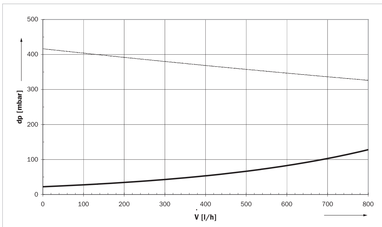
Fig. 30: Curva della perdita di pressione del circuito secondario
