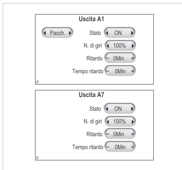
Fig. 23: Determinazione del numero di giri minimo
