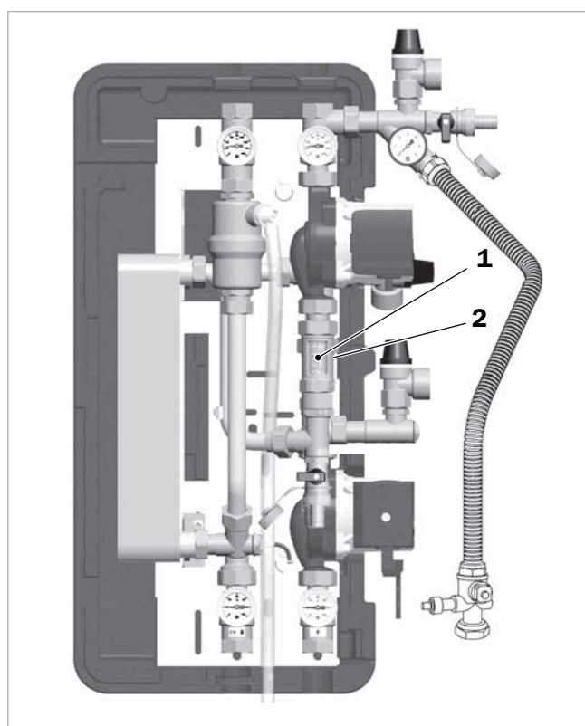
Fig. 17: Posizione delle valvole di compensazione
