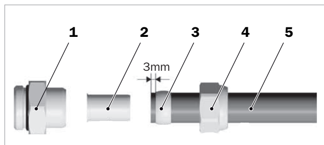
Fig.3: Montaggio del collegamento a vite con anello di bloccaggio
