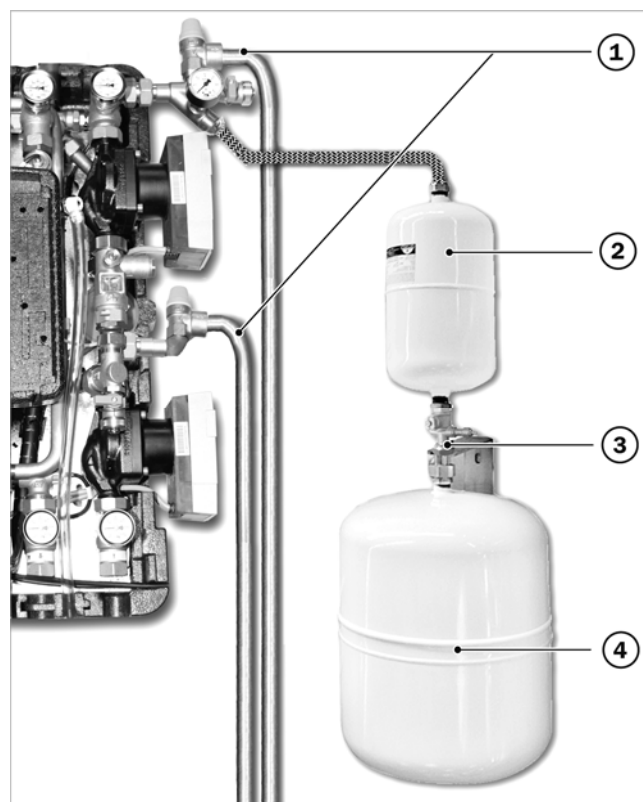
Fig.2: Vaso di espansione solare (qui: SOL-24) e vaso addizionale solare montati
