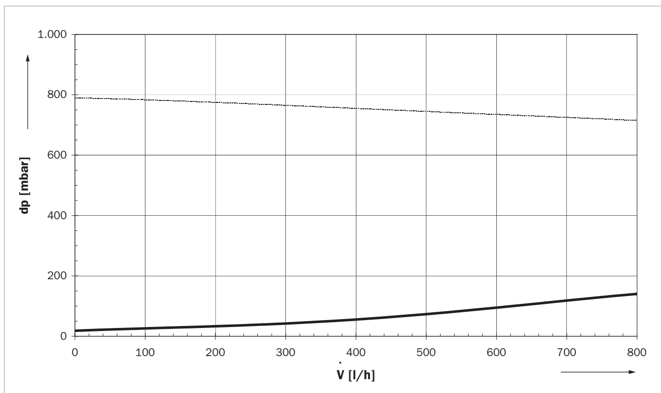
Fig. 29: Curva della perdita di pressione del circuito primario
