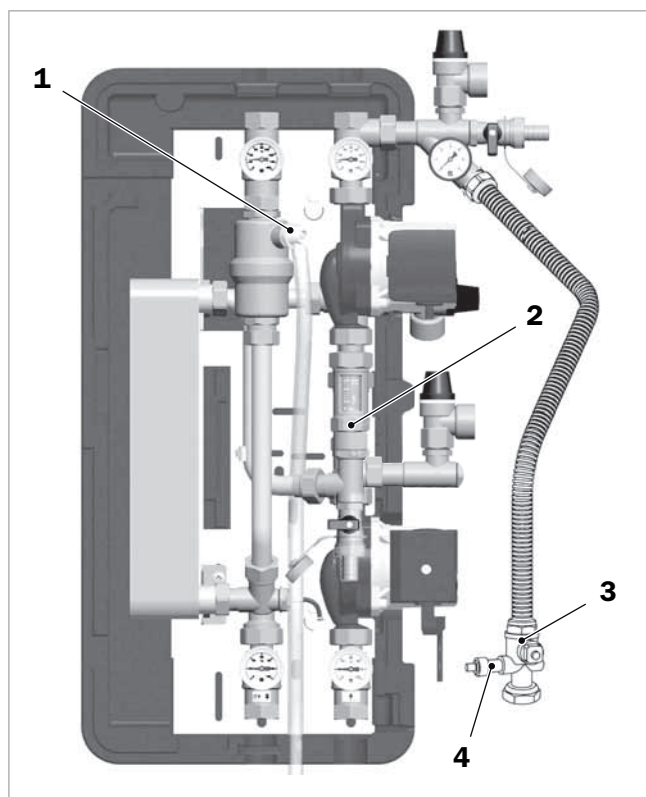
Fig. 25: Posizione delle valvole per la manutenzione
