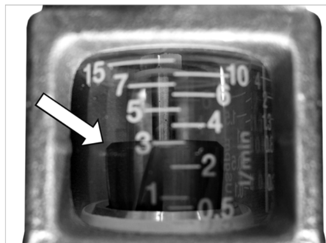
Fig. 18: Lettura del flusso volumetrico nel bordo superiore del galleggiante (qui 3 l/min.)
