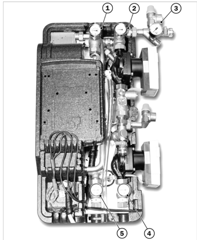
Afb. 1: overdrukventielen gemonteerd
