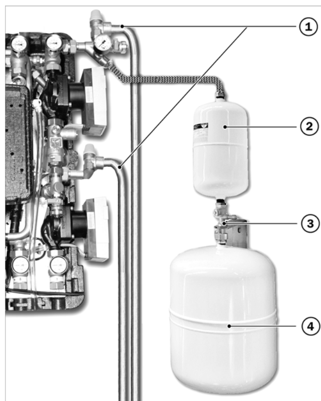
Afb.2: zonnestelsysteem-expansie- (hier: SOL-24) en voorschakelvat gemonteerd
