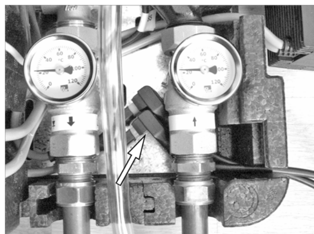
Afb. 5: Molex-stekkers verbinden
