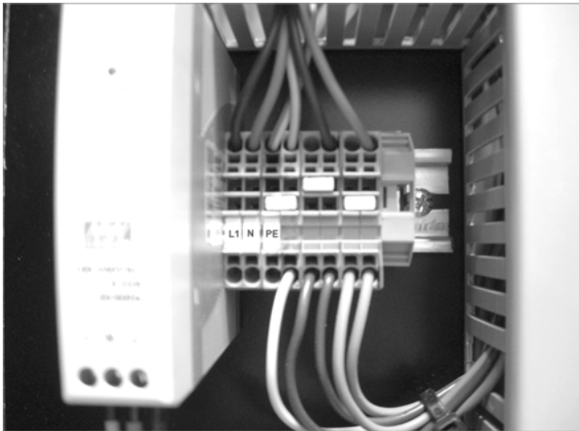
Abb. 3: Spannungsversorgung anschließen
