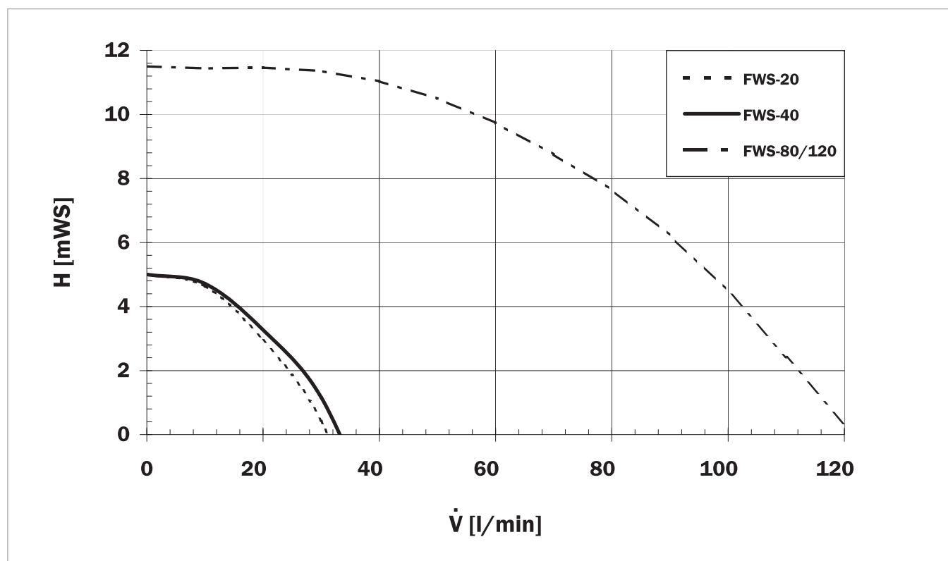
Abb. 4: Externe Restförderhöhe Trinkwasser-Zirkulation
