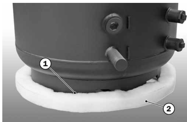
Abb. 6: Isolierschal um den Speicherfuß legen
