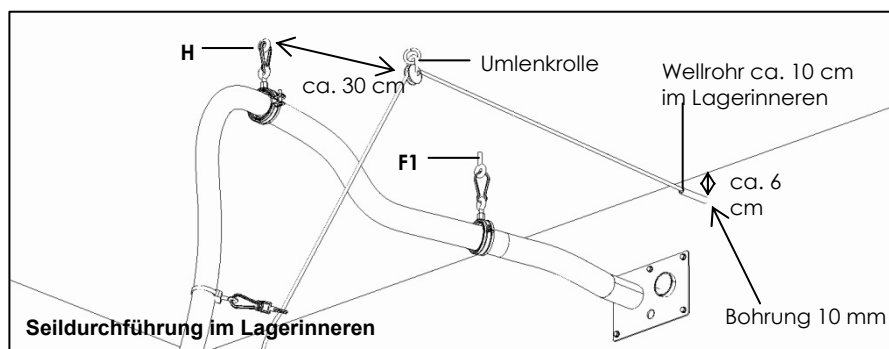
Bauteil: Umlenkrolle
