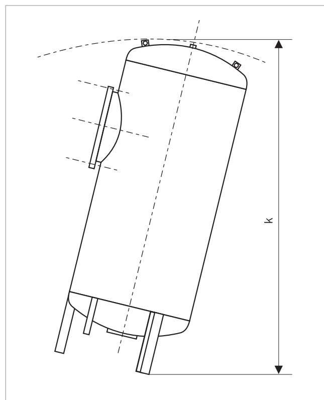
Abb. 105: Kippmaß
