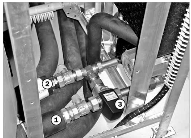
Abb. 43: Warmwasserverrohrung anschließen
