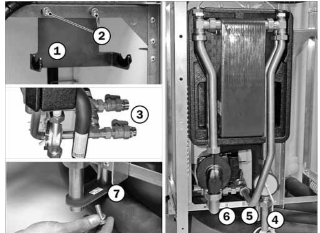
Abb. 42: Montage der Warmwasserstation
