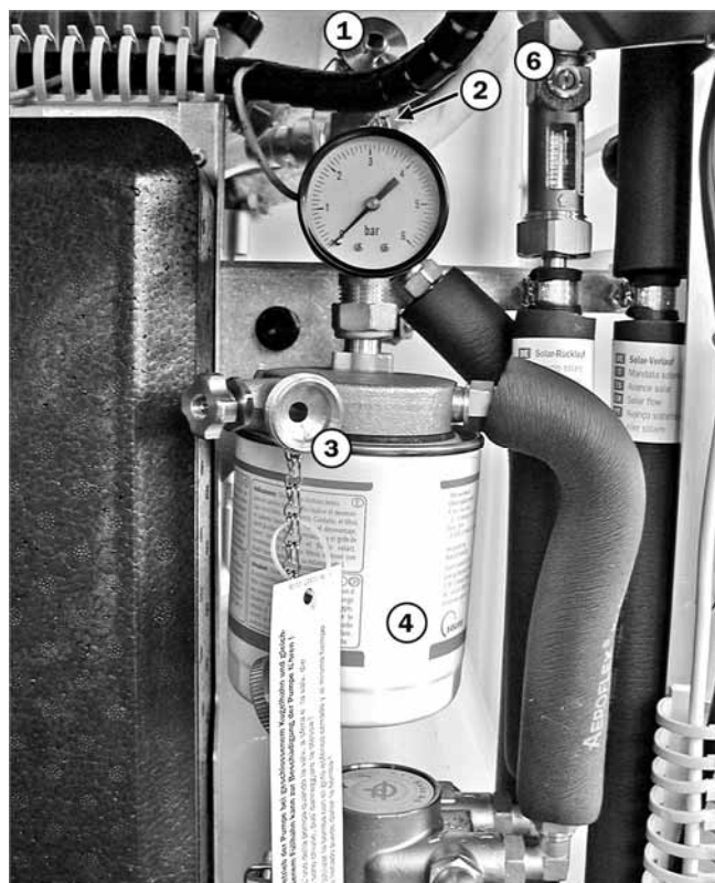
Abb. 96: Solarkreis Komponenten
