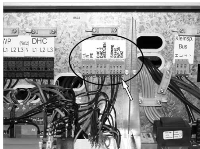
Abb. 54: Platine Steuerleitung
