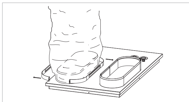
Abb. 30: Schlauch befestigen
