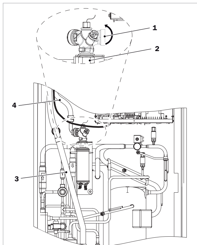
Abb. 23: Anschlussstutzen drehen
