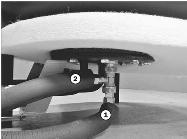
Abb. 40: Solarleitungen am Solar-Wärmeübertrager montieren
