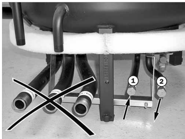
Abb. 97: Spülanschlüsse Solar-Wärmeübertrager
