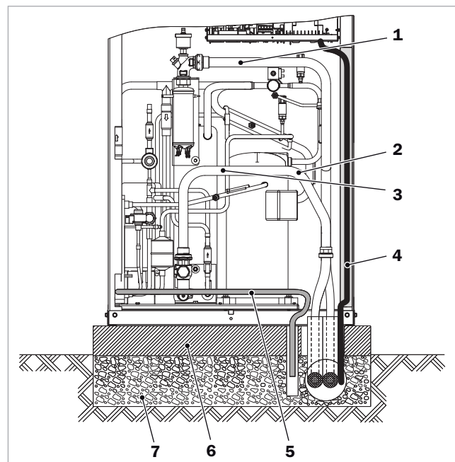
Abb. 21: Versorgungsleitungen
