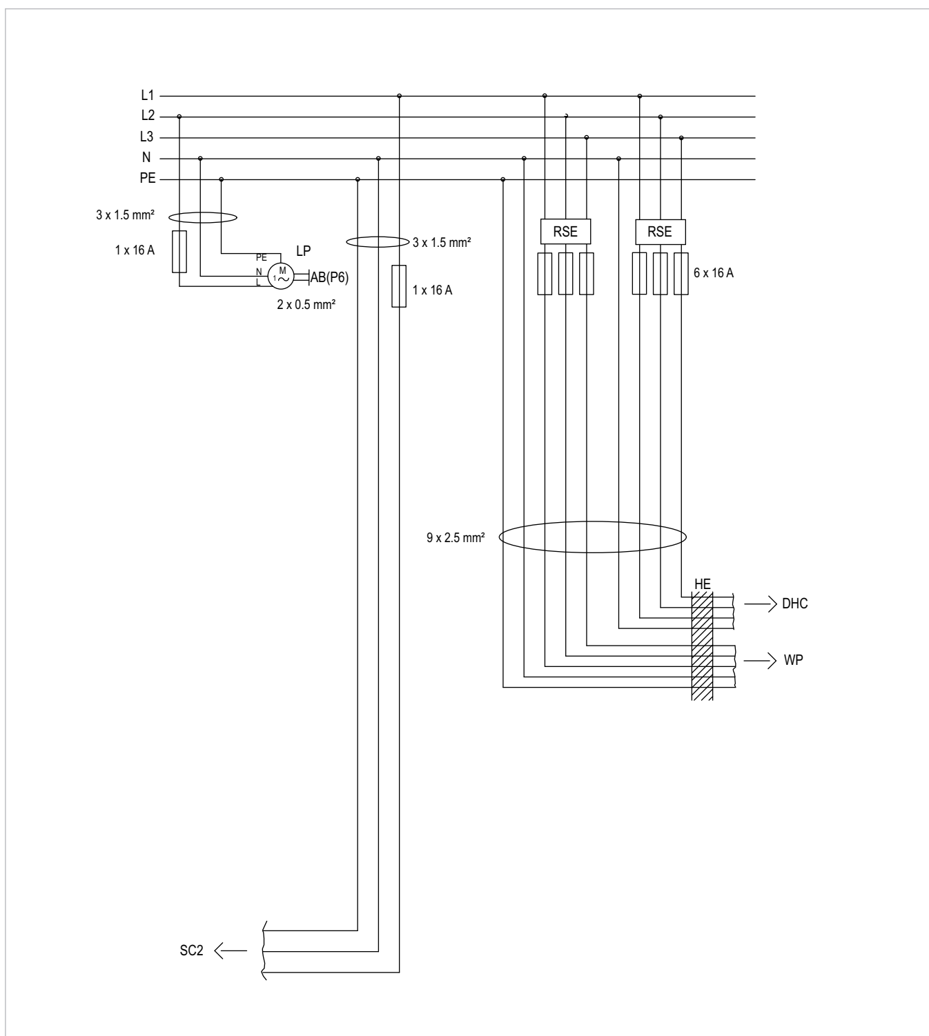
Abb. 115: Stromanschluss
