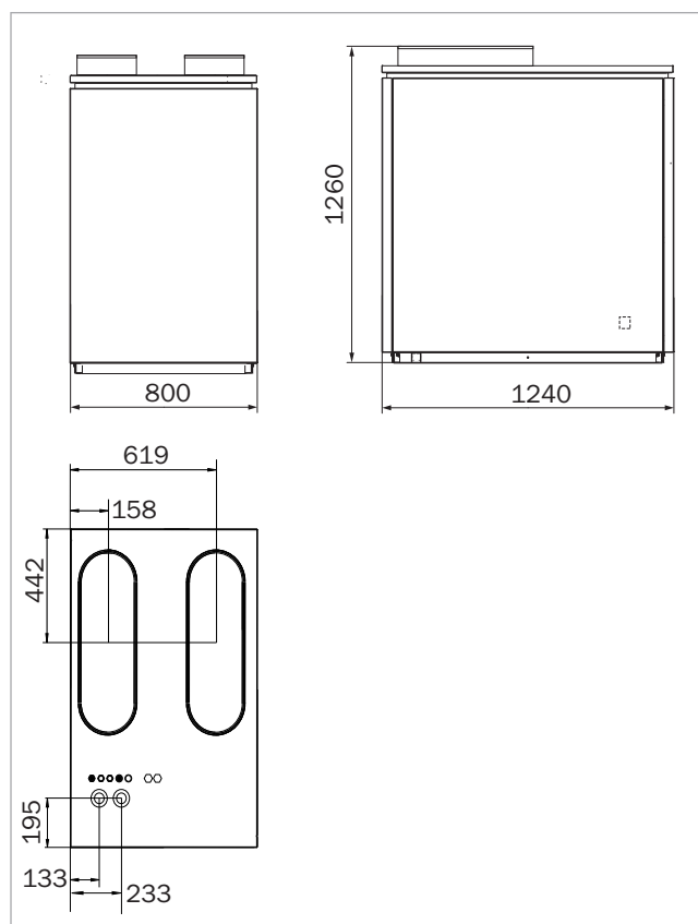
Abb. 101: SolvisVaero I, Maße in mm
