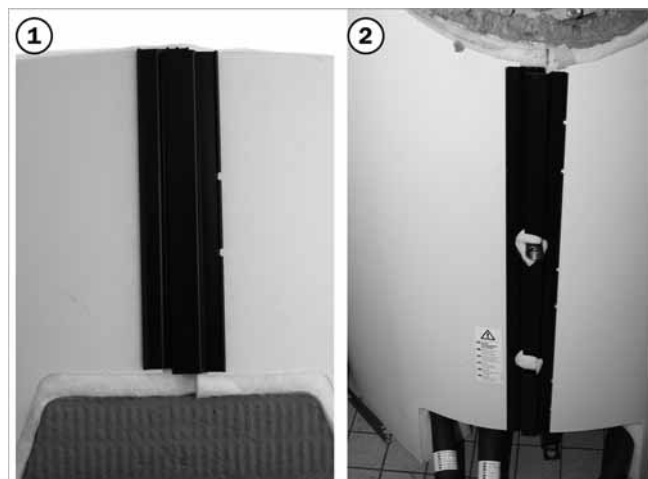
Abb. 73: Isolierung oben (1) und unten (2) schließen
