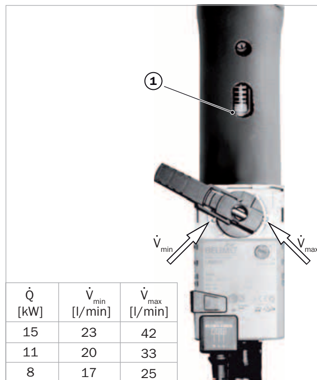
Abb. 64: Durchfluss einstellen
