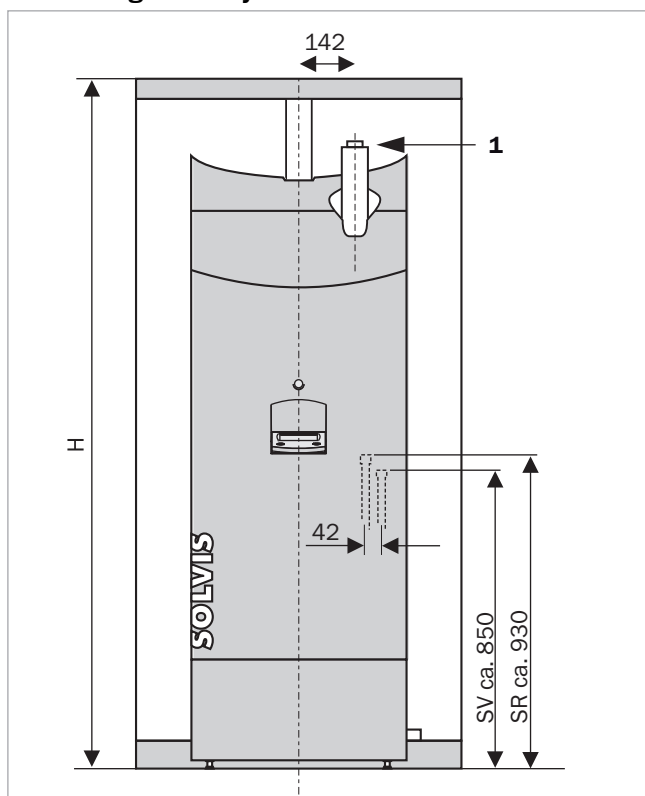
Abb. 102: Frontansicht, 1 Optionaler Austritt, Maße in mm
