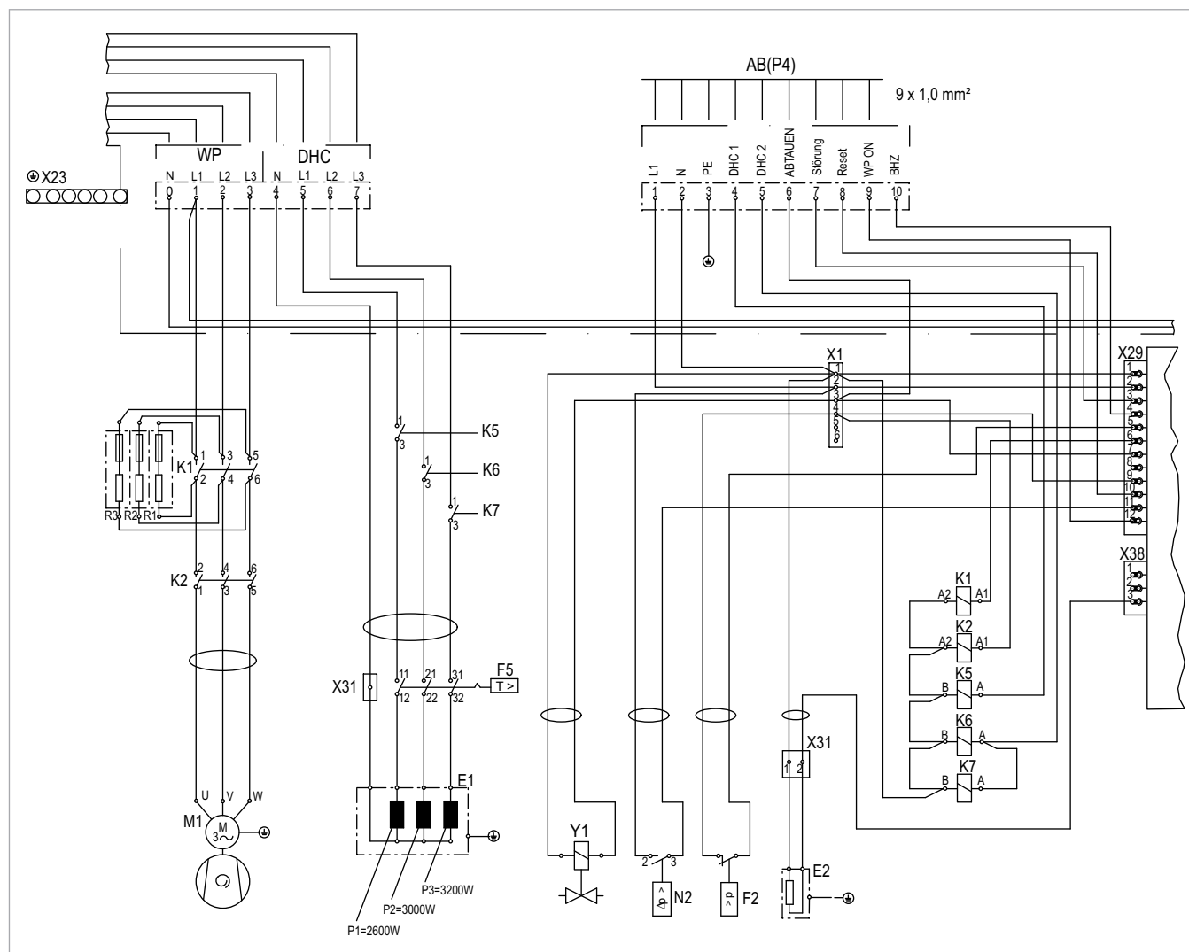
Abb. 116: Integrierte Wärmepumpen-Steuerung (IWS), Netzspannungsseite
