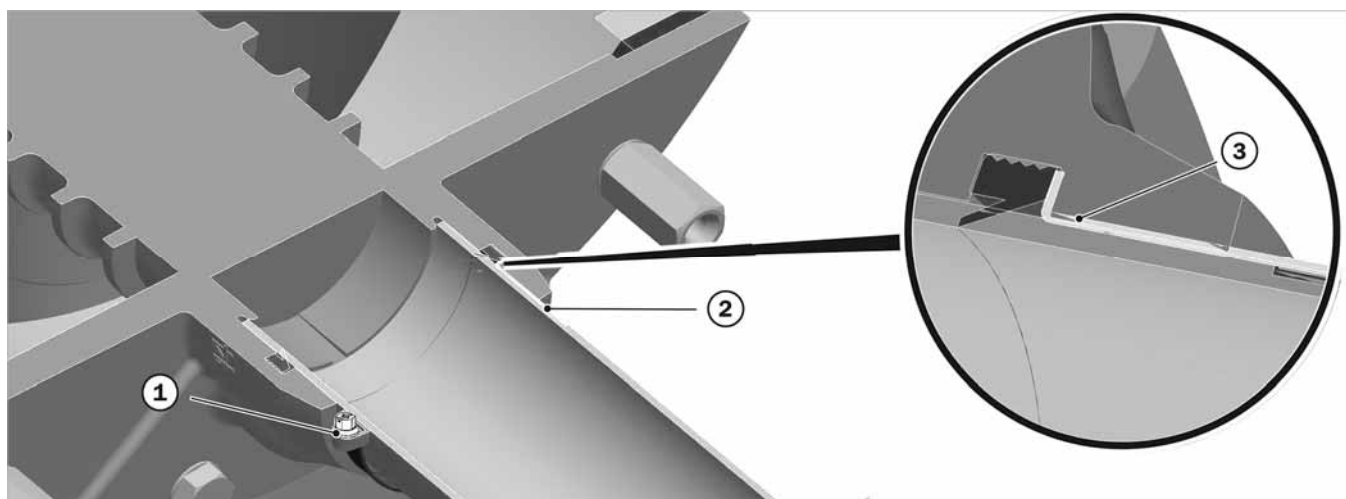
Abb. 2: Schnitt durch Abgasbogen / Cross section of exhaust elbow / Sezione attraverso la curva della tubazione fumi / Corte del codo de salida de humos / Vista seccionada do cotovelo de gás de escape / Coupe du coude d'évacuation des gaz / Doorsnede door rookgasbochtstuk
