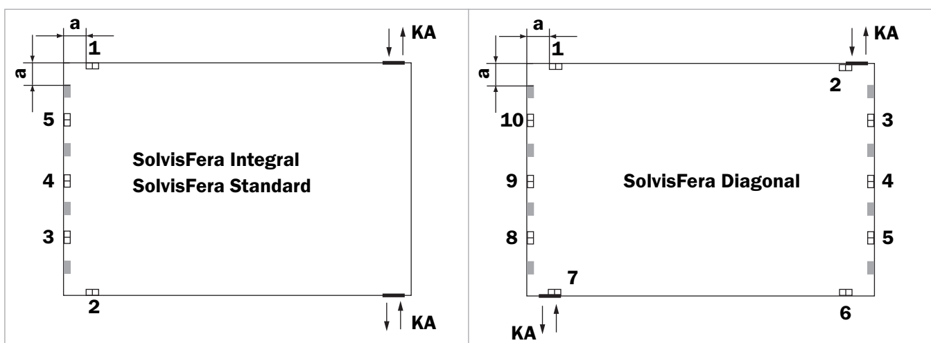
Abb. 1: Draufsicht / Vista dall'alto / Vista superior
