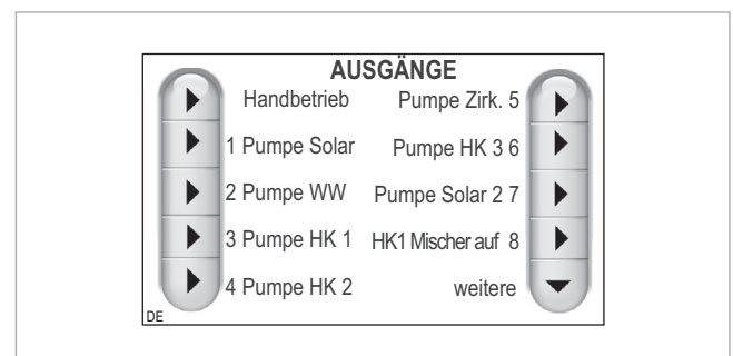
Abb. 13: Das Menü „Ausgänge“
