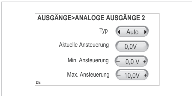
Abb. 15: Menü des Analogausgangs O-2
