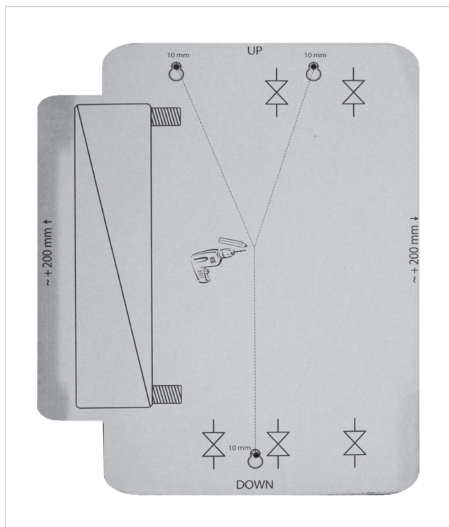
Abb. 1: Bohrschablone SÜS-50-HE / SÜS-90-HE
