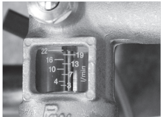
Abb. 18: Volumenstrom an oberer Kante des Schwebekörpers ablesen
