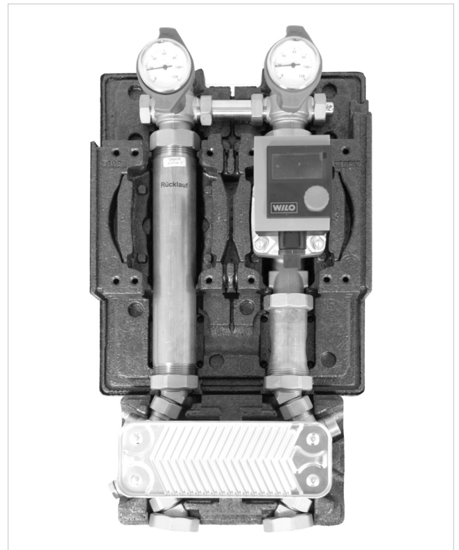
Abb. 11: HK-WÜT montiert
