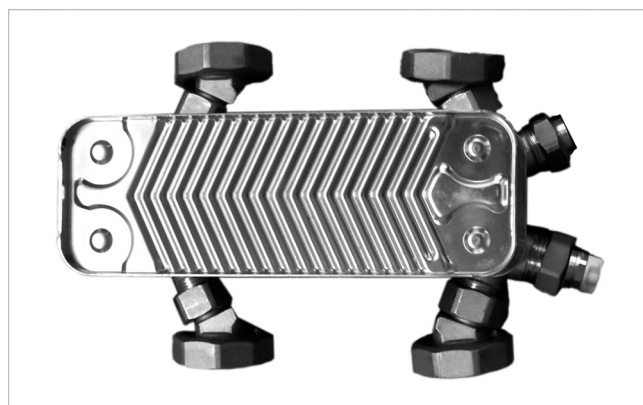
Abb. 1: Platten-Wärmeübertrager
