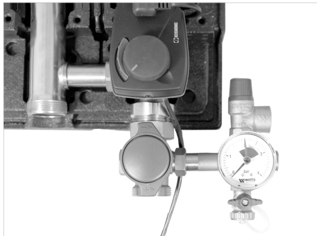
Abb. 14: Sicherheitsgruppe, montiert
