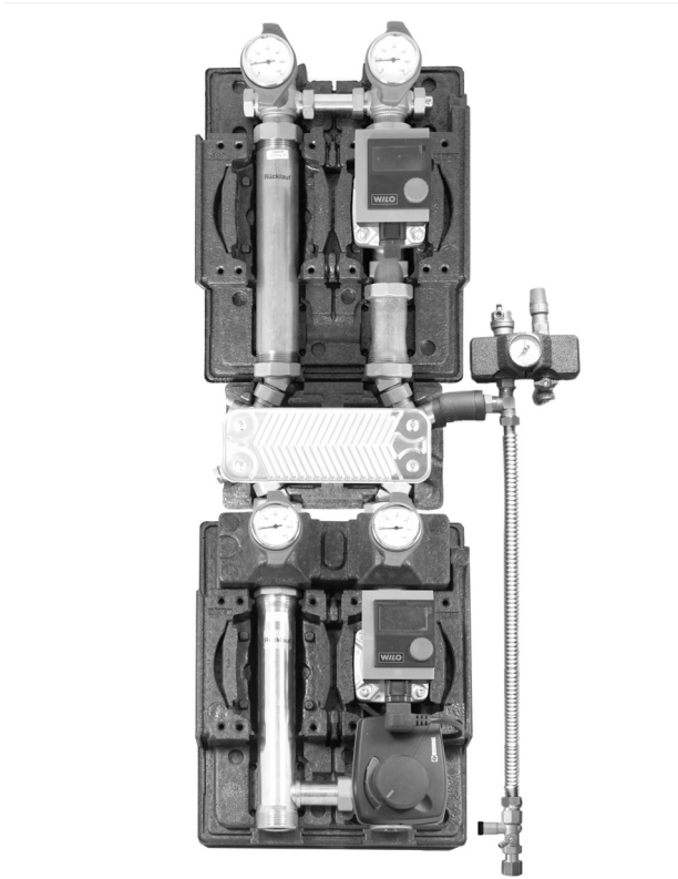
Abb. 13: HK-STS montiert
