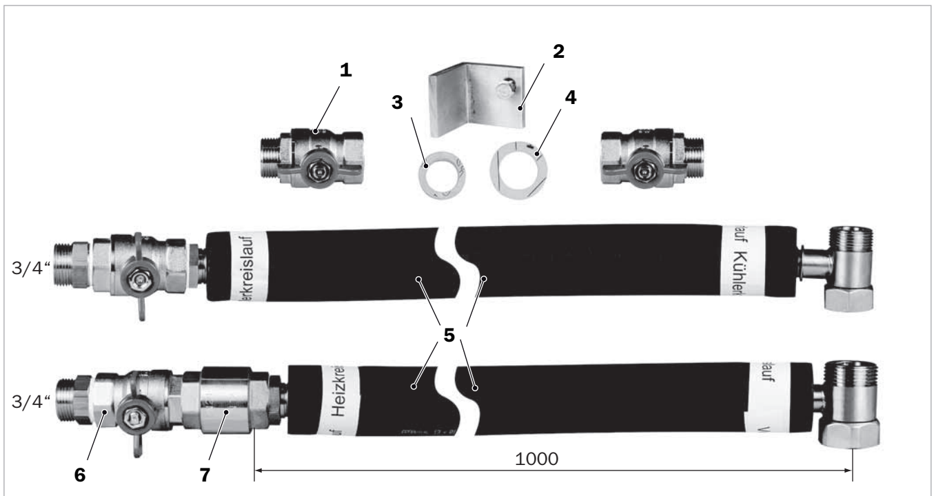
Abb. 1: Anschlusssatz zur Anbindung von Solartrocknern an Solvis-Schichtenspeichern
