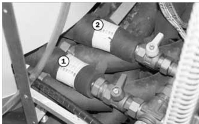
Abb. 3: Kugelhähne geschlossen
