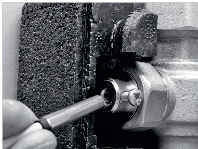
Fig. 3: Montaje del sensor de temperatura de retorno
