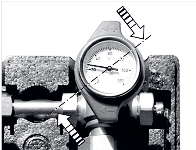
Afb. 4: Kogelkraan met geïntegreerde thermometer
