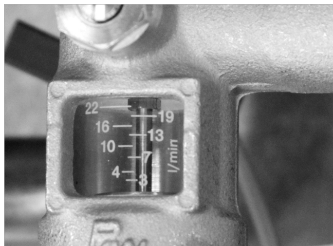
Fig. 18: Lectura del caudal volumétrico en el borde superior del cuerpo flotante
