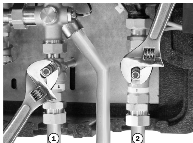
Afb. 8: kogelkranen half geopend / geheel geopend
