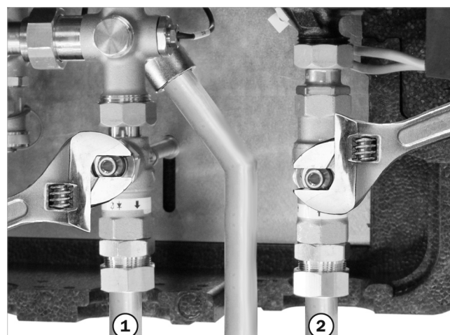
Afb. 7: kogelkranen gesloten
