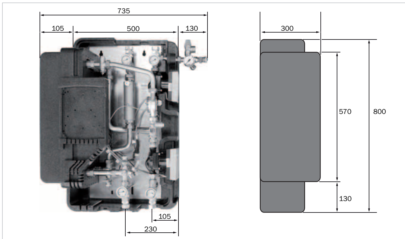
Afb. 24: afmetingen van de zonnewarmte-overdrachtgroep
