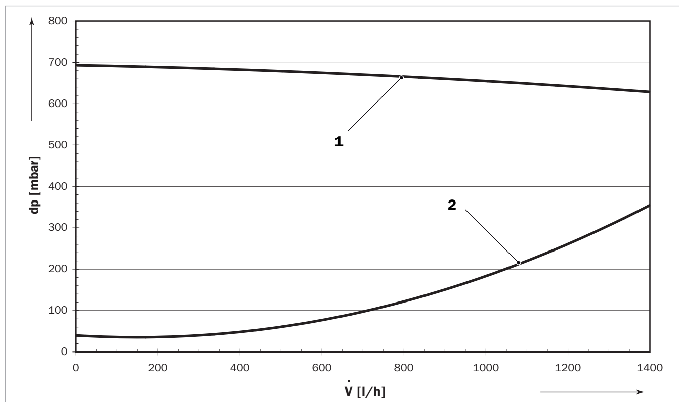
Afb. 26: drukverlieskromme van het secundair circuit
