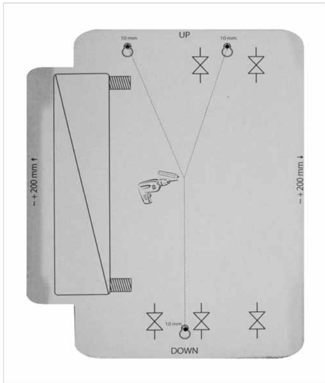
Afb. 1: boorsjabloon SÜS-50-HE / SÜS-90-HE
