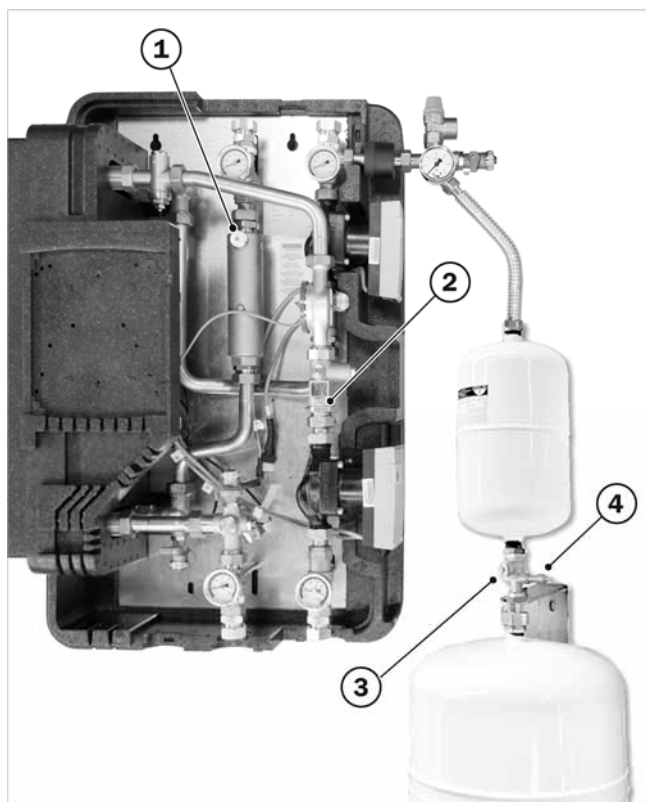
Afb. 23: positie van de ventielen/kleppen voor het onderhoud
