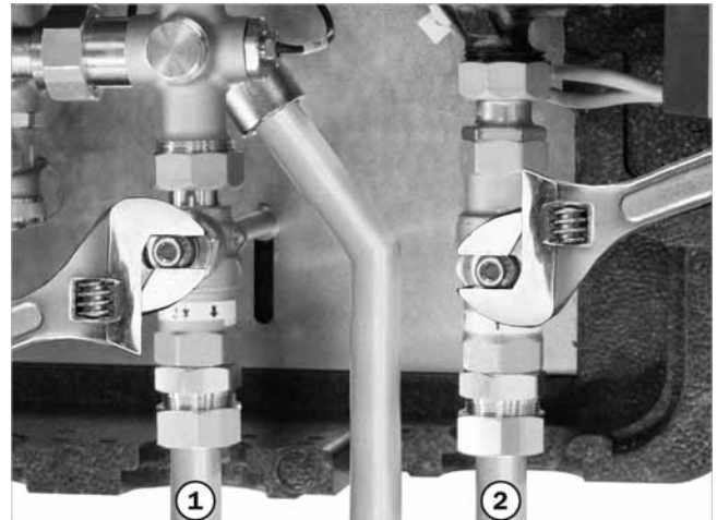
Afb. 7: kogelkranen gesloten
