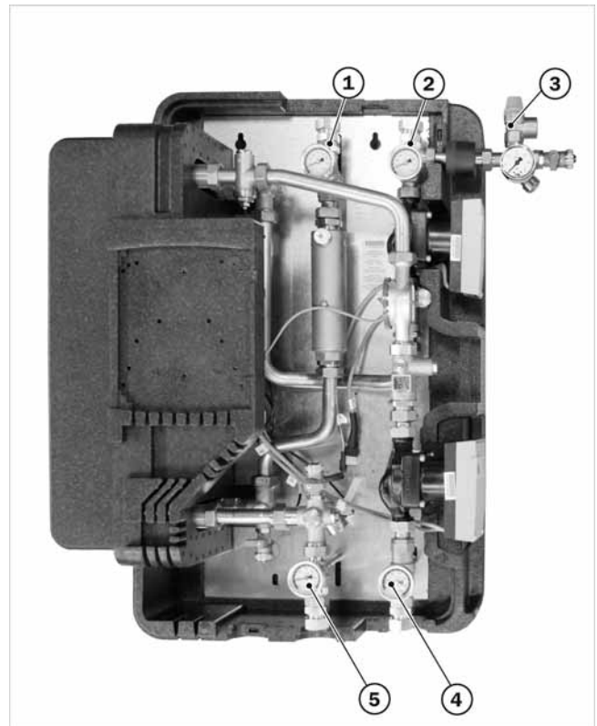
Afb. 2: overdrukventielen gemonteerd
