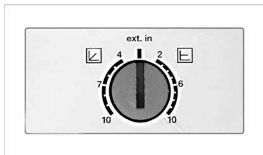
Afb. 12: pomp op „ext. in“ instellen
