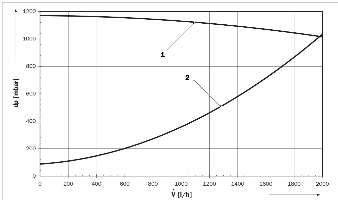
Afb. 25: drukverlieskromme van het primair circuit
