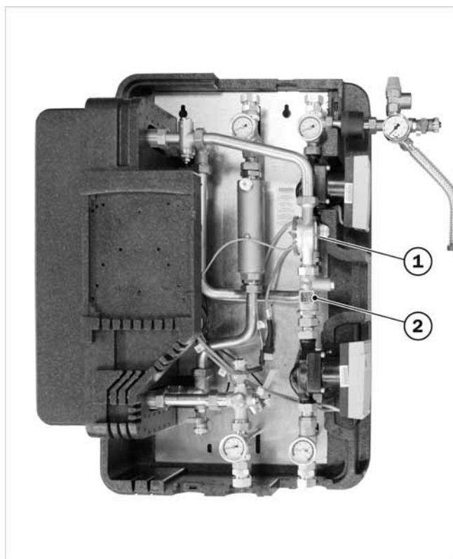
Afb. 17: positie van de flowmeters
