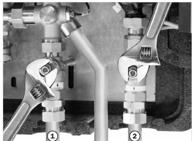
Afb. 8: kogelkranen half geopend / geheel geopend
