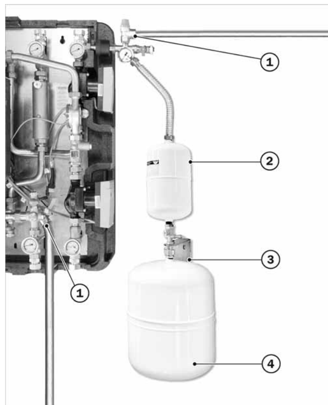
Afb.3: zonnestelsysteem-expansie- (hier: SOL-24) en voorschakelvat gemonteerd
