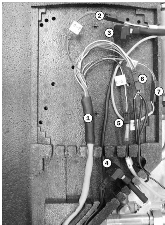
Afb. 5: aansluitingen op de verlengkabel
