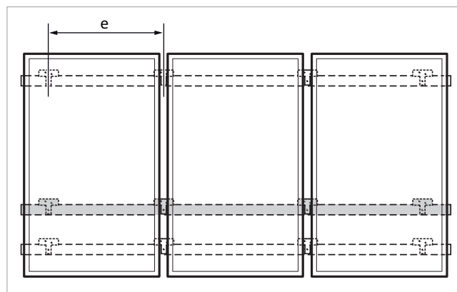
Abb. 11: Zusätzliche Halteschiene (Nebeneinandermontage)
