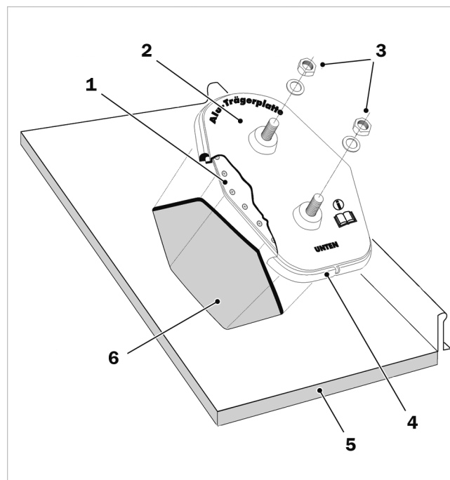
Fig. 19: Montagem à face do telhado
