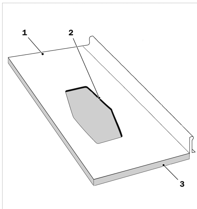
Afb. 26: Uitsparing uitsluitend in het plaatwerk maken
