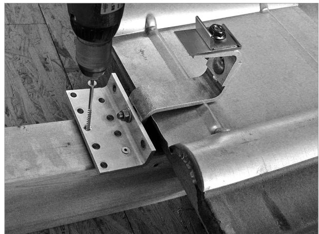
Abb. 1: Aufdachhalter befestigen
