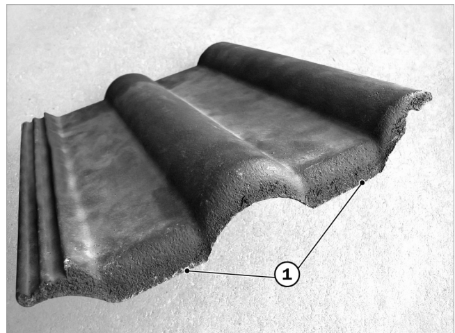
Abb. 2: Fußverfaltung am Dachziegel
