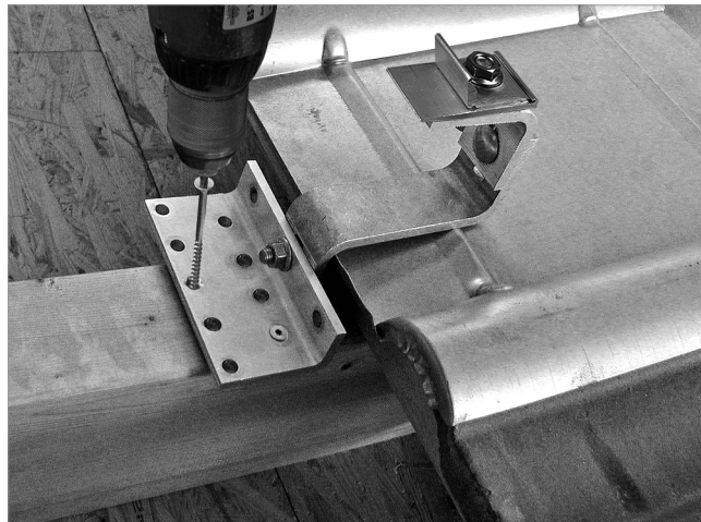
Fig. 9: Fixar o suporte de telhado
