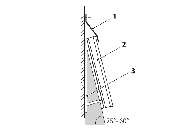
Abb. 10: Kollektor mit Abdeckblech
