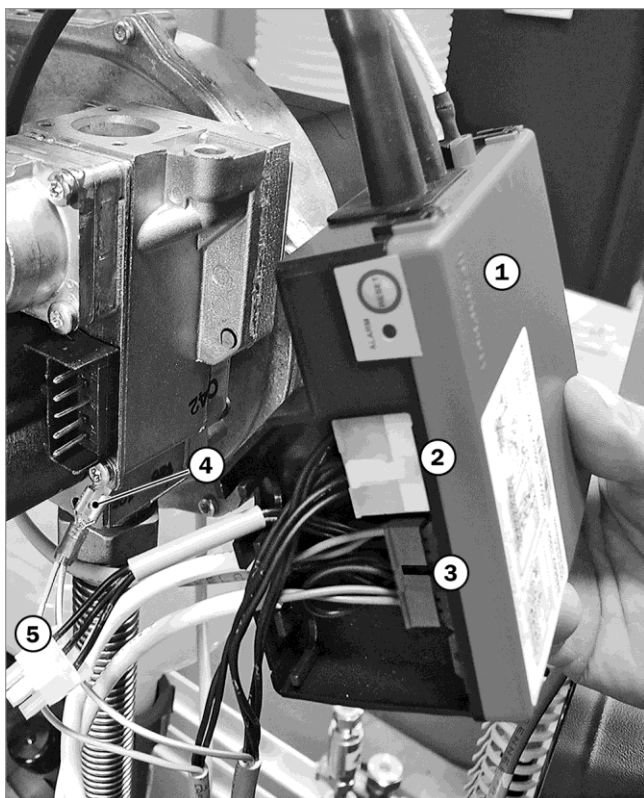
Abb. 15: Feuerungsautomat anschließen
