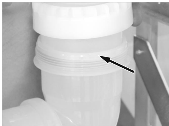
Abb. 10: Abgasbogen gerade ausgerichtet verschrauben
