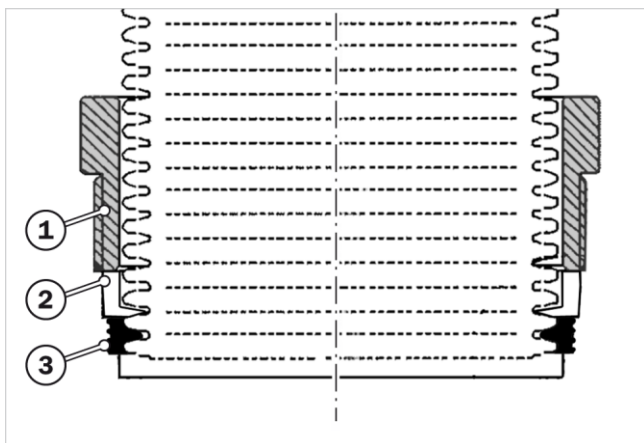
Abb. 8: Verschraubung aufgesteckt
