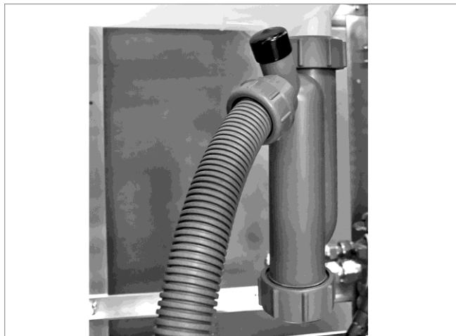
Abb. 12: Siphon mit Kondensatschlauch montieren
