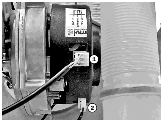
Abb. 22: Gebläse anschließen
