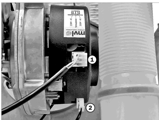
Abb. 16: Gebläse anschließen
