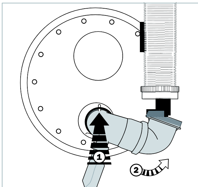
Abb. 9: Abgasbogen montieren
