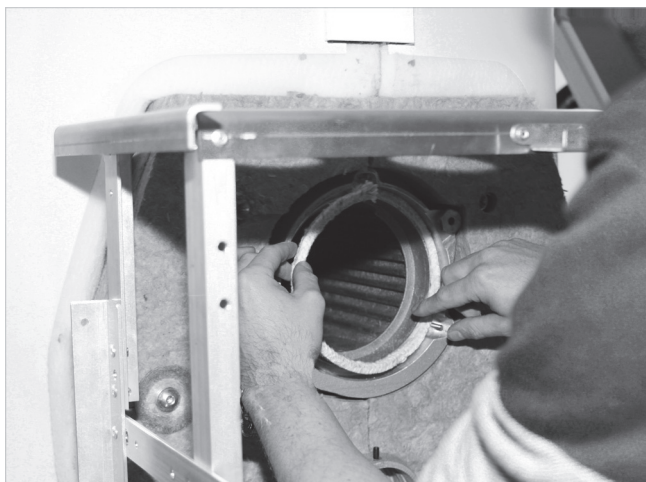
Abb. 1: Brennerdichtschnur einlegen
