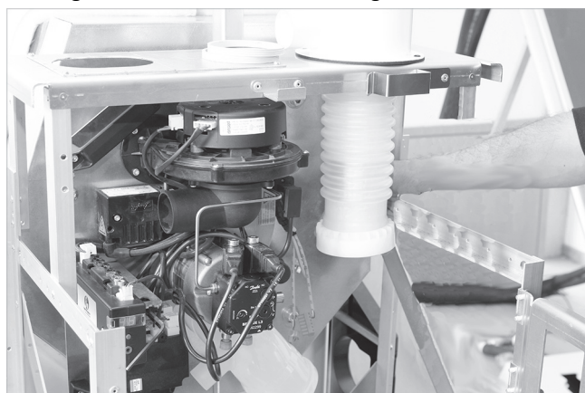
Abb. 13: Abgasanschlusstück gerade ausrichten
