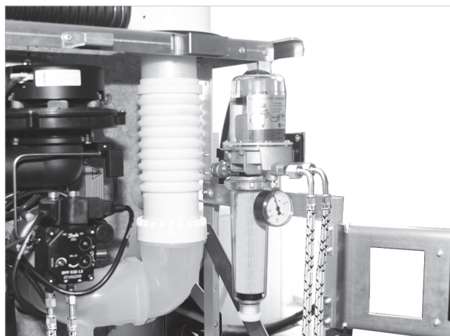
Abb. 18: Ölleitungen anschließen
