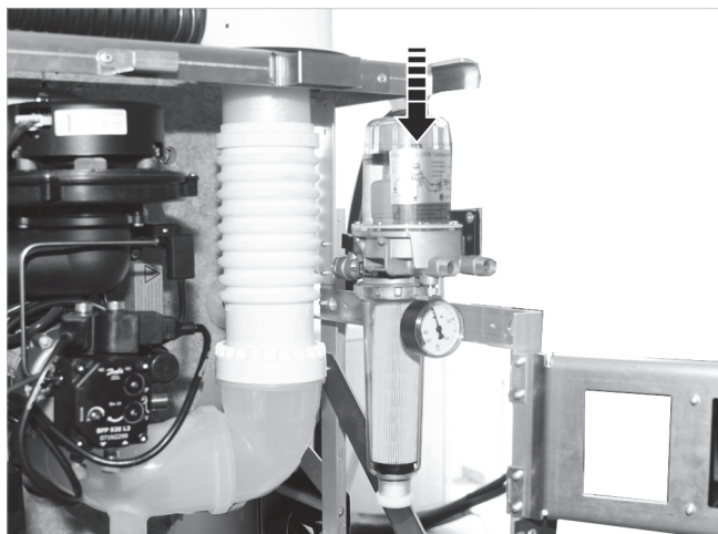
Abb. 17: Ölfilter aufgesteckt
