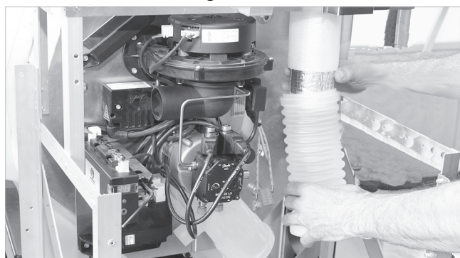
Abb. 12: Abgasanschlusstück aufstecken
