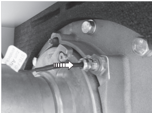
Abb. 20: mSTB einstecken
