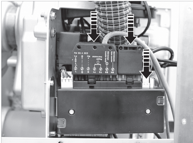
Abb. 23: Stecker aufstecken
