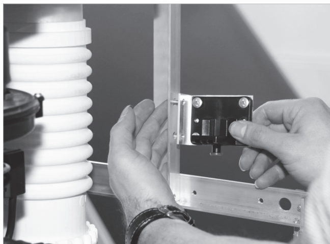
Abb. 16: Ölfilter-Halterung befestigen
