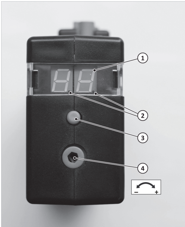
Abb. 28: Gebläsedrehzahl am Interface einstellen
