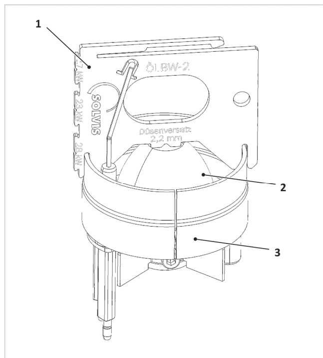
Abb. 35: Mischkopf mit aufgesetzter Einstelllehre
