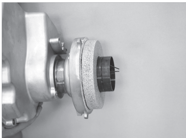
Abb. 5: Kesseltürstein aufsetzen
