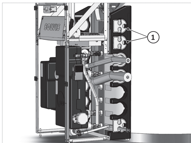
Abb. 19: Ölleitung durch Dreierreduzierung führen
