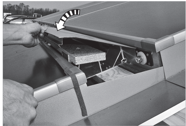
Abb. 69: Erstes Zwischenblech in Nut eindrehen, aufsetzen und andrücken
