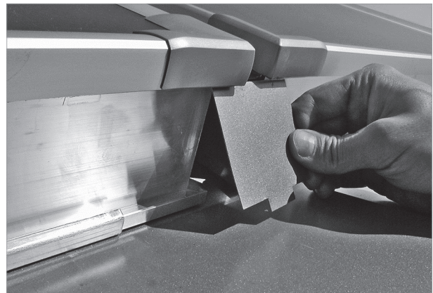
Abb. 88: Die kleinen Bleche vor die Zwischenräume der Kollektoren setzen
