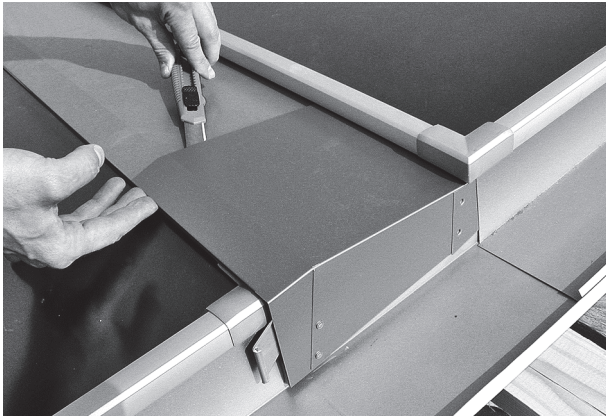
Abb. 76: Bei nachträglichem Zugang: Klebeverbindung zwischen den Blechen lösen ...
