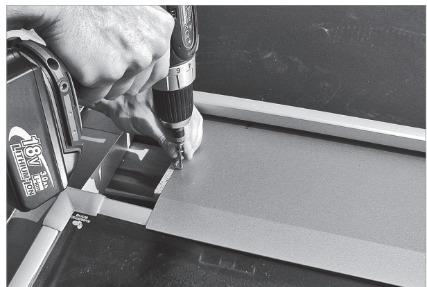
Abb. 71: Zwischenblech etwa 10 mm von linker Außenkante anschrauben
