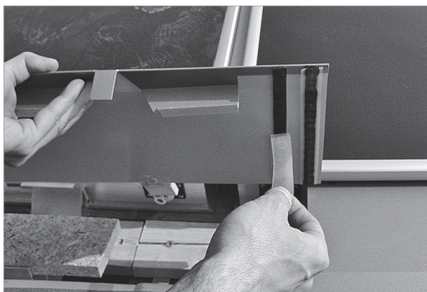
Abb. 72: An der Unterseite des Kreuzungsbleches Schutzstreifen abziehen
