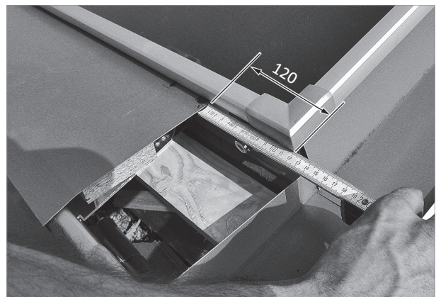
Abb. 70: Blech auf Abstand zur Außenkante bringen
