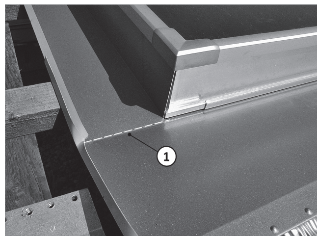
Abb. 57: Unterer Seitenblech bis zum Knick nach unten schieben
