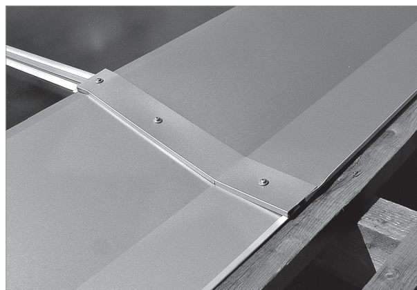
Abb. 82: Das obere Blech mit dem unteren Blech verschrauben
