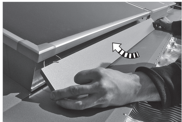
Abb. 89: Die langen Verkleidungsbleche vor die Stirnseite der Kollektoren setzen
