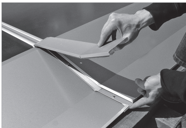
Abb. 81: Das obere Blech des Verbinders mit dem unteren in Deckung bringen
