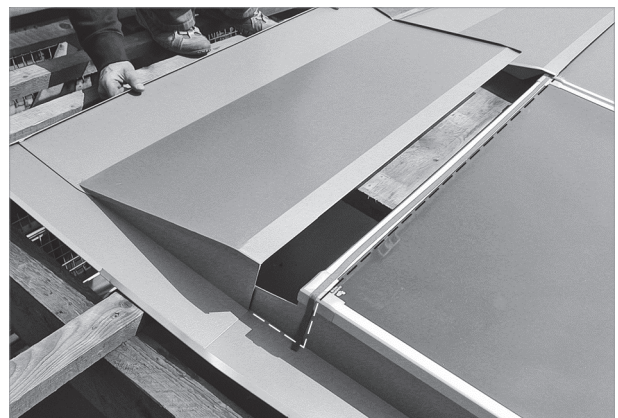
Abb. 79: Oberblech auf das Seitenblech aufsetzen und gegen den Kollektor schieben
