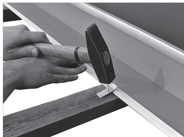
Abb. 66: Bleche mit Blechhaften an Dachlatten fixieren
