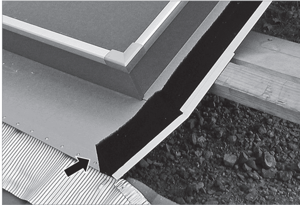
Abb. 85: Flugschneekeile aufgeklebt
