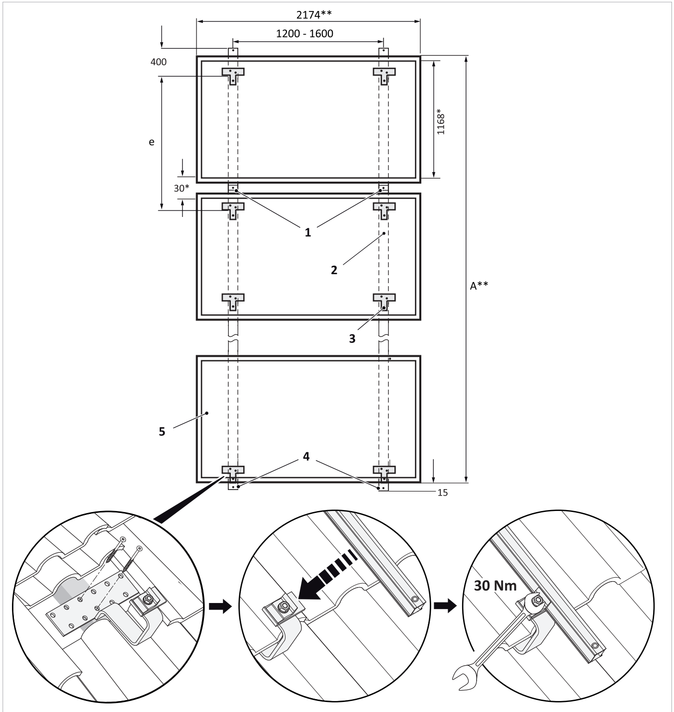
Abb. 19: Übereinandermontage der Dachhalter und Montageschienen.
