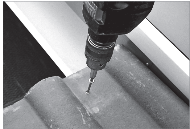
Abb. 87: Ziegel neben dem Seitenblech befestigen
