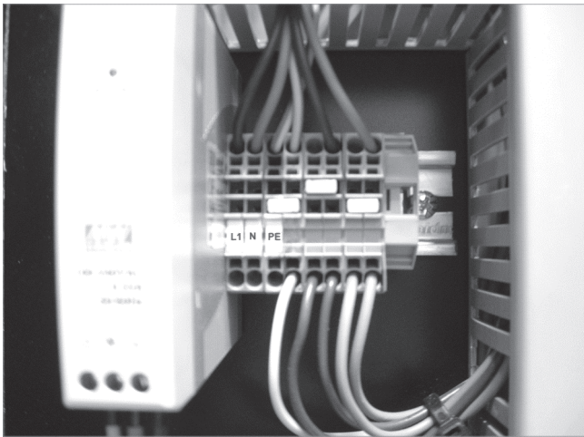
Abb. 3: Spannungsversorgung anschließen
