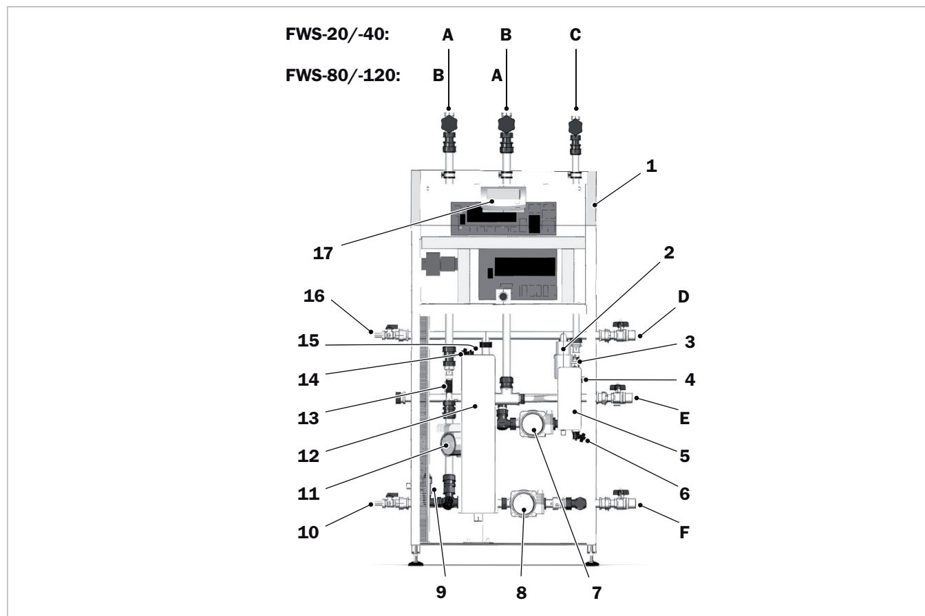
Abb. 2: Frischwasserstation
