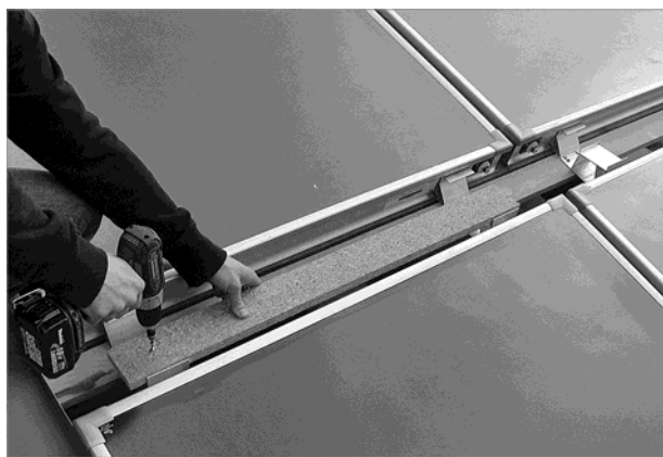
Fig. 67: Atornillar los apoyos de la chapa intermedia a los distanciadores de colectores
