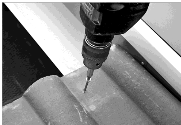
Fig. 87: Fijar la teja junto a la chapa lateral
