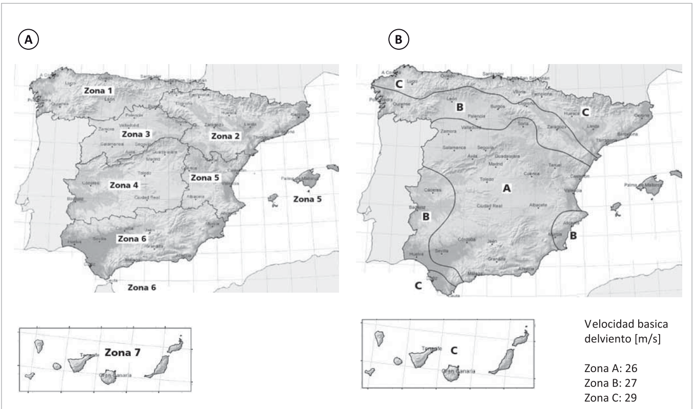
Fig. 99: Distribución de zonas de carga de nieve y de viento en España A zonas de carga de nieve
