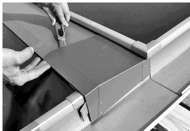
Fig. 76: En caso de acceso posterior: soltar la unión adhesiva entre las chapas ...
