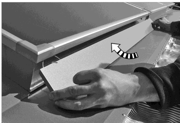
Fig. 89: Colocar las chapas de revestimiento largas delante el lado frontal de los colectores
