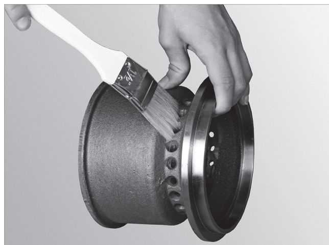
Abb. 145: Konus mit Pinsel reinigen
