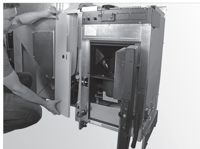
Abb. 79: Verkleidung vorne einhängen
