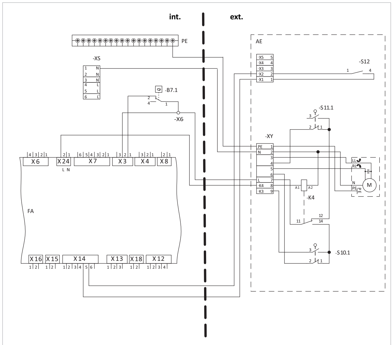
Abb. 189: Anschlussplan Absperreinheit
