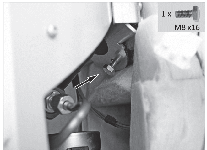
Abb. 33: Vorratsbehälter festschrauben
