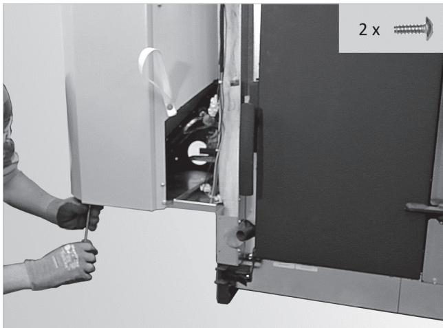
Abb. 31: Zwei Stück Schrauben entfernen
