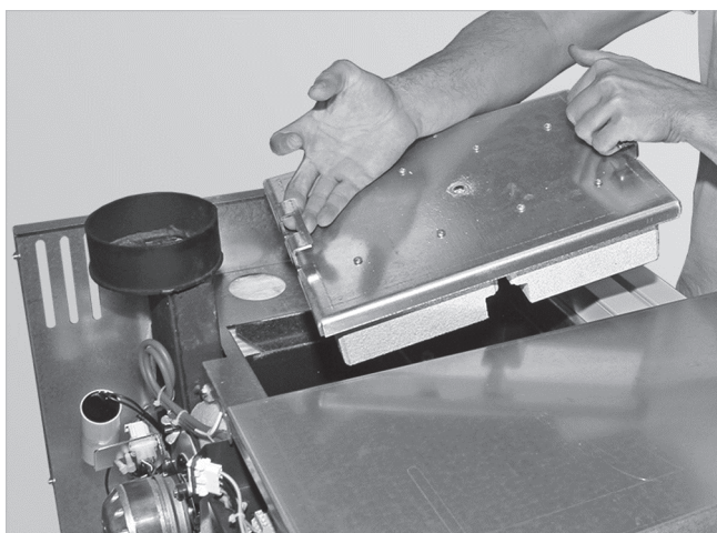
Abb. 19: Deckel abnehmen
