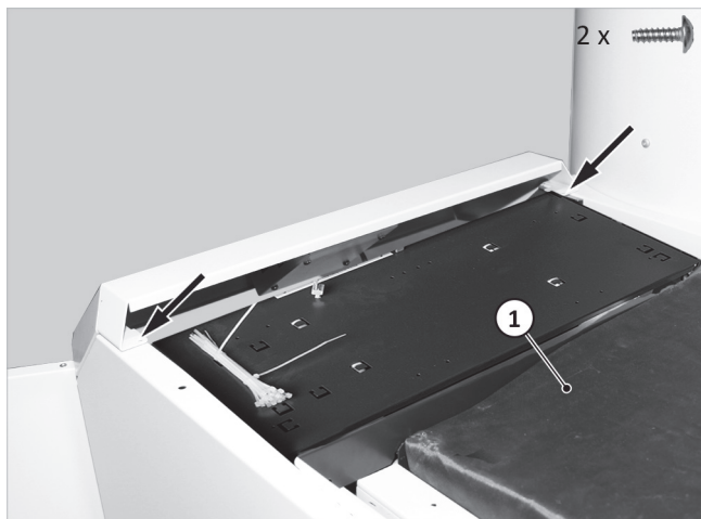
Abb. 94: Schalterblende befestigen, Isolierung auflegen
