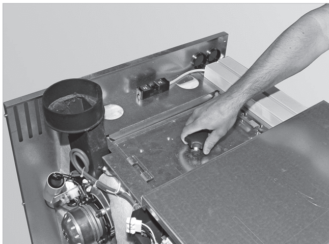
Abb. 18: Verschraubung entfernen
