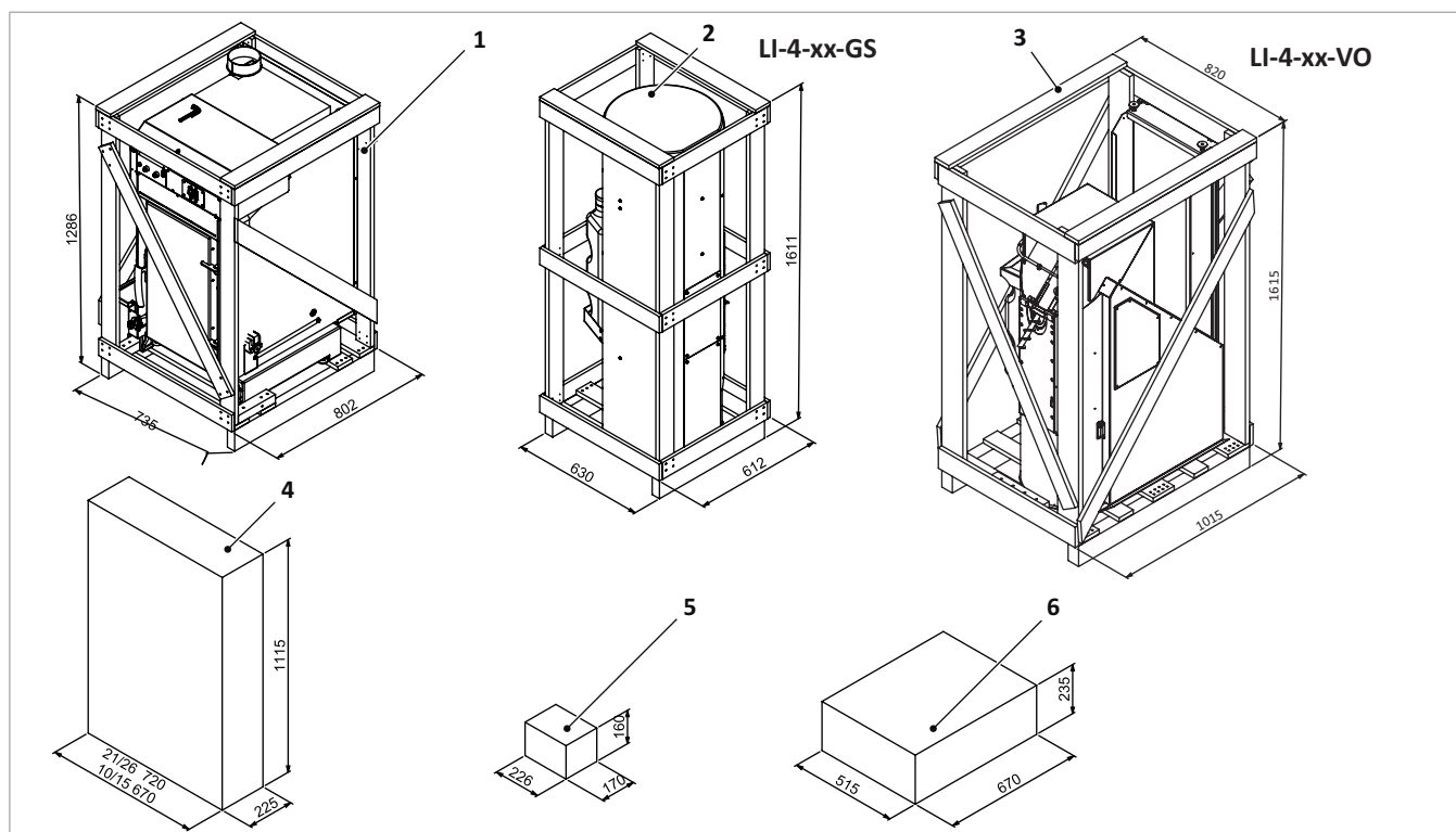
Abb. 4: Lieferumfang SolvisLino 4
