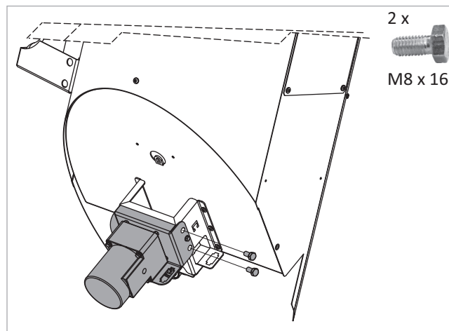
Abb. 63: Schneckenmotor anschrauben
