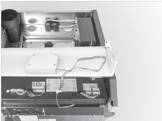
Abb. 93: Kabel zusammenstecken
