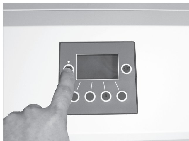
Abb. 127: SolvisLino ausschalten
