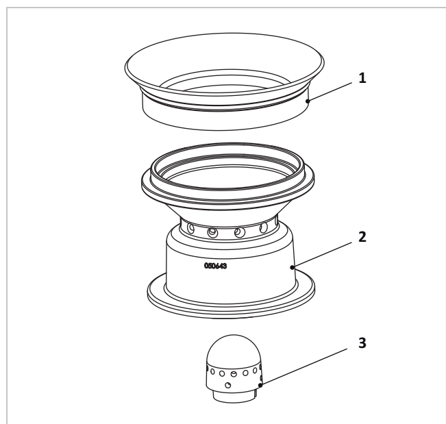
Abb. 152: Zusammenbau Brennertopf
