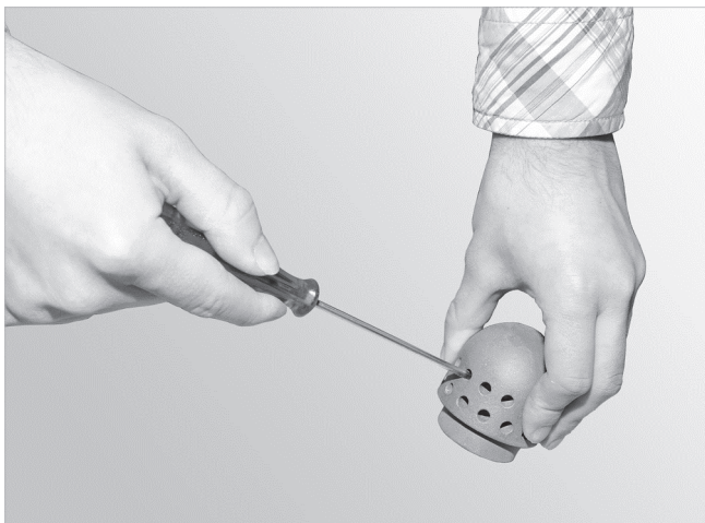
Abb. 149: Primärluftdorn vorsichtig reinigen
