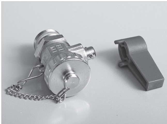
Abb. 26: Griff bei Füll- und Entleerhahn abziehen
