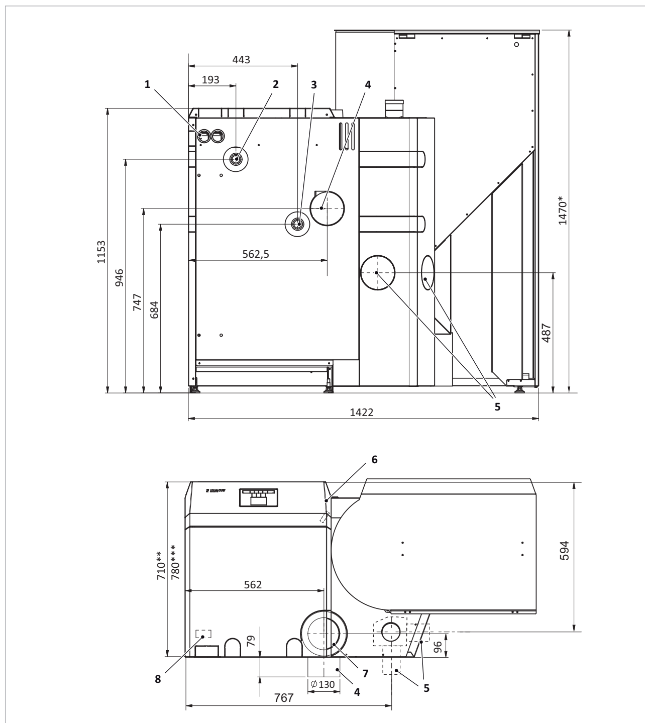
Abb. 179: Ansichten SolvisLino 4 mit Vorratsbehälter (LI-4-xx-VO)
