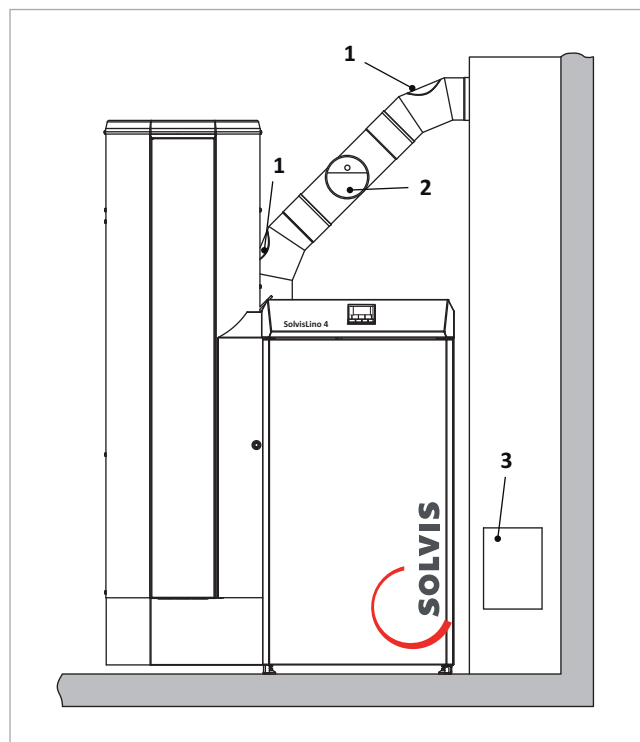
Abb. 161: Reinigungsöffnungen (Ansicht ohne Isolierung)
