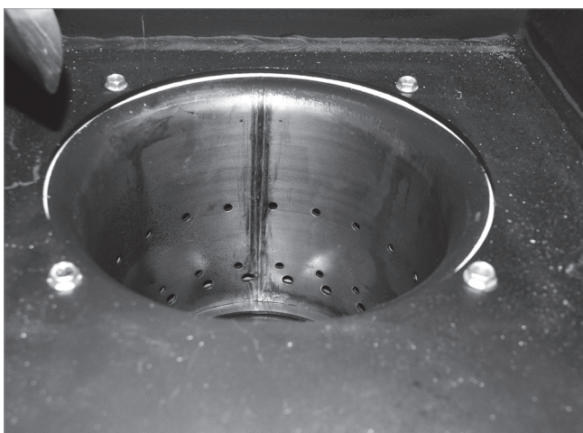
Abb. 150: Sekundärluftlöcher im Brennertopf reinigen
