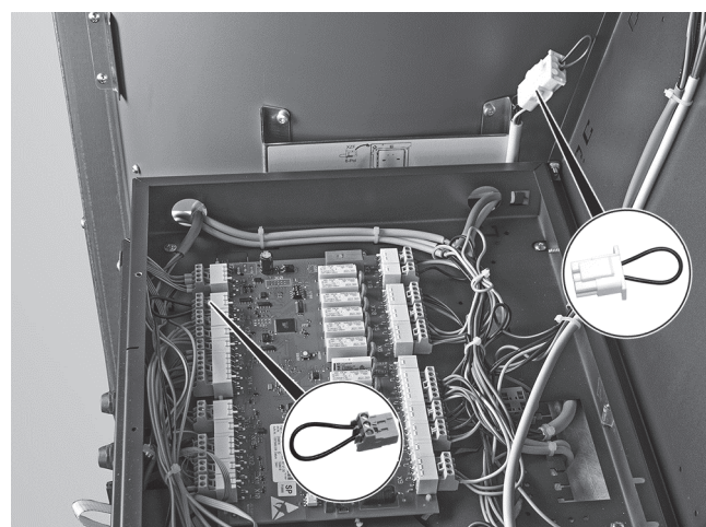
Abb. 70: Stecker anstecken
