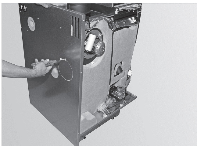
Abb. 20: Vorstanzung ausbrechen
