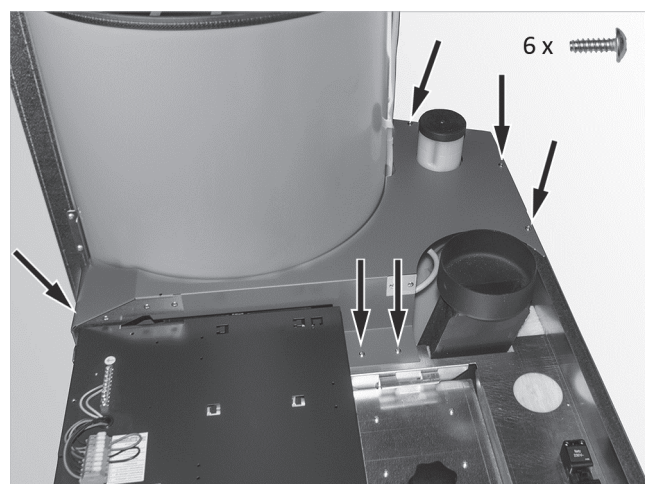
Abb. 78: Verkleidung befestigen
