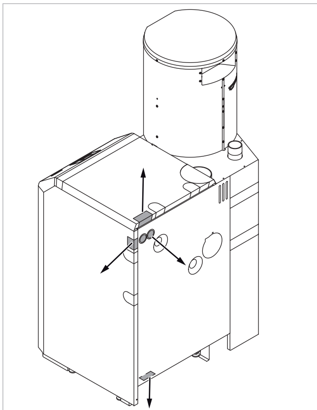
Abb. 115: Kabeldurchführungen – Ansicht von hinten
