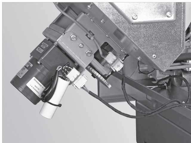
Abb. 65: Stecker anstecken
