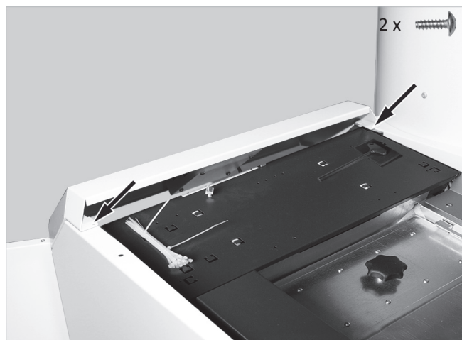
Abb. 111: Beide Schrauben an Schalterblende lösen
