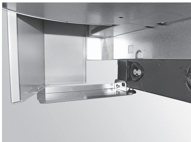
Abb. 100: Sockel für Aschebehälter einhängen
