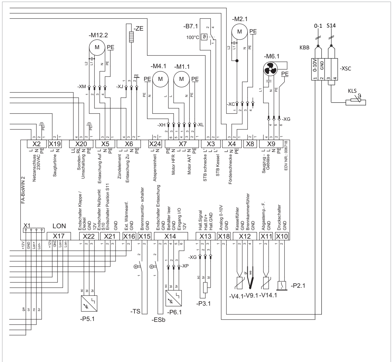
Abb. 185: Grundschaltbild SolvisLino 4 (Teil 2)
