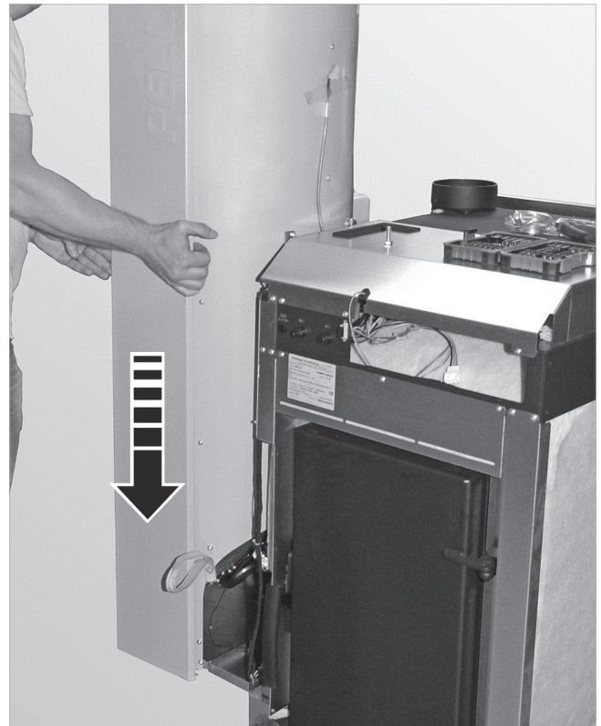
Abb. 32: Blende abnehmen
