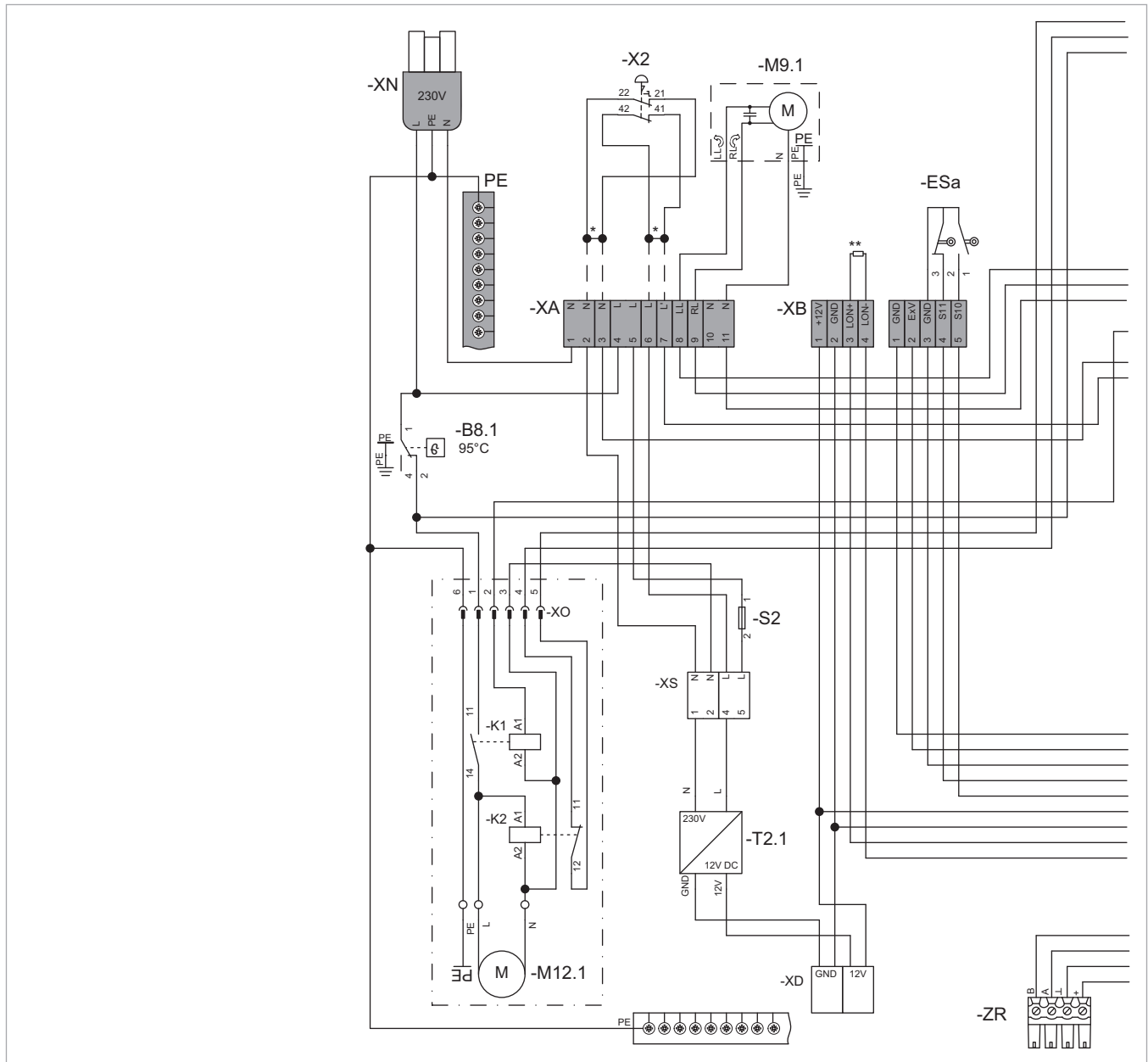
Abb. 184: Grundsaltbild SolvisLino 4 (Teil 1)
