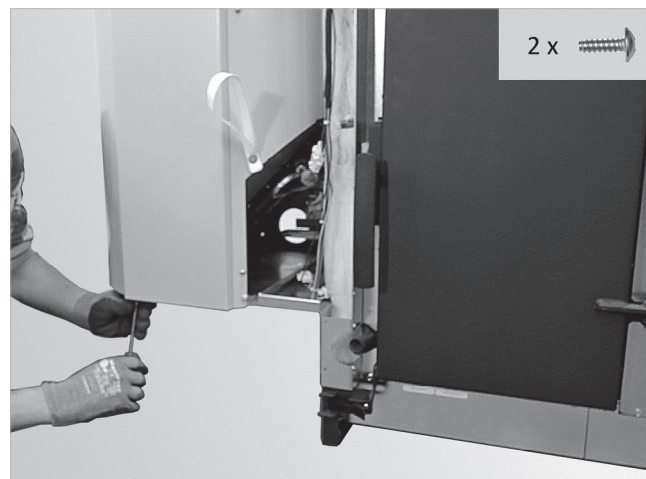
Abb. 39: Blende befestigen
