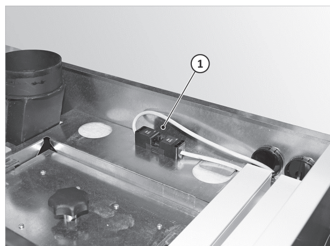
Abb. 174: Stecker prüfen
