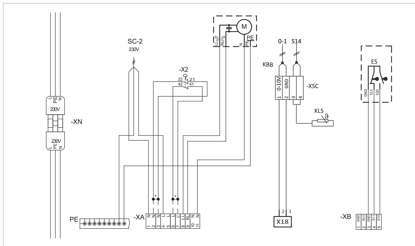
Abb. 186: Anschlussplan Umschalteneinheit
