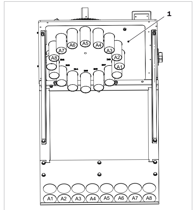
Abb. 53: Förderschläuche A1 bis A8 auf Umschalteneinheit montieren - Ansicht von unten
