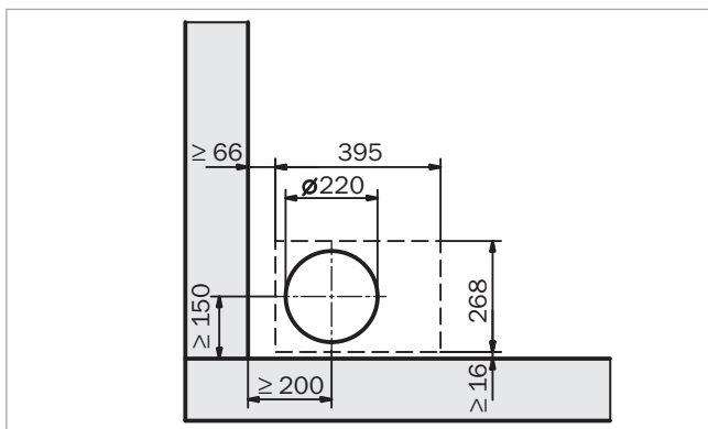
Abb. 11: Mauerdurchführung für Umschalteinheit, Wand links – Vorderansicht
