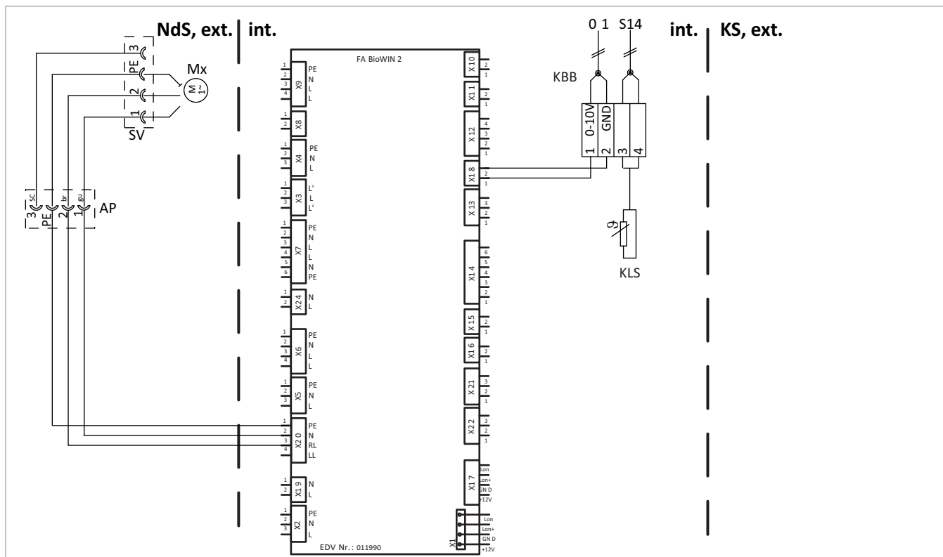
Abb. 95: Anschlussplan Maulwurfentnahme
