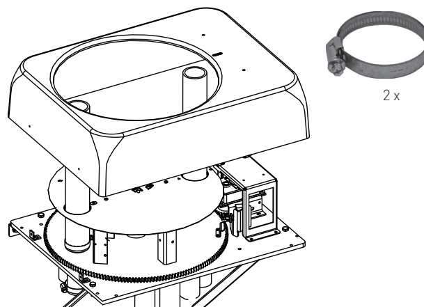
Abb. 57: Förder- und Rückluftschlauch anschließen (Abb. der Umschalteinheit ohne Brandschutzmanschetten)
