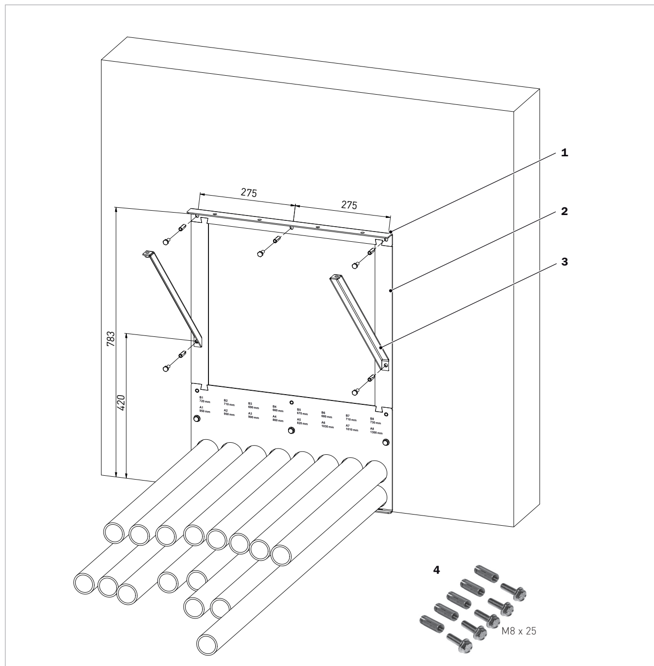
Abb. 47: Montagewinkel, Verbinder und Abstützwinkel montieren
