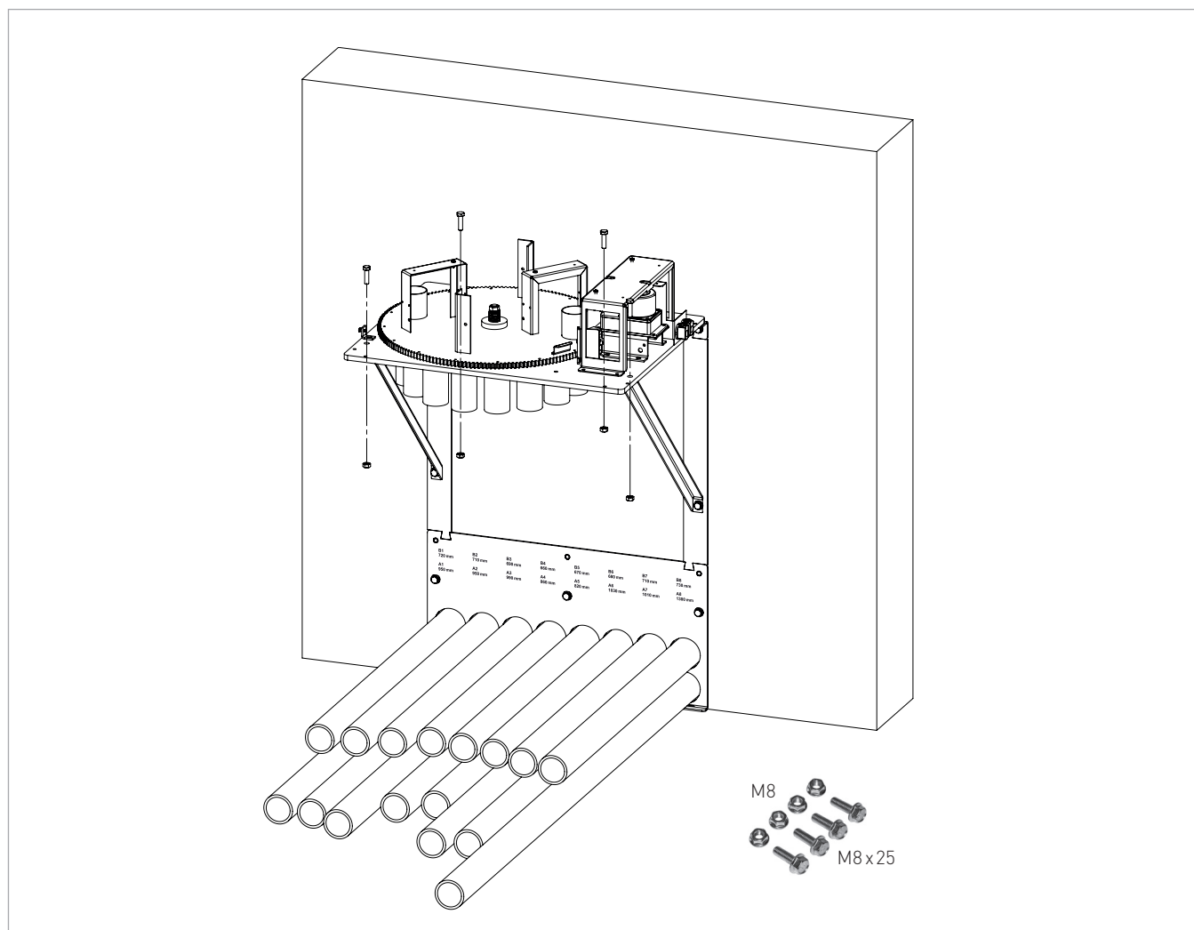
Abb. 48: Umschalteinheit montieren
