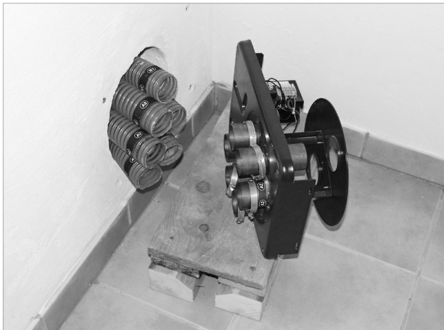
Abb. 15: Umschalteneinheit mit Schlauchenden
