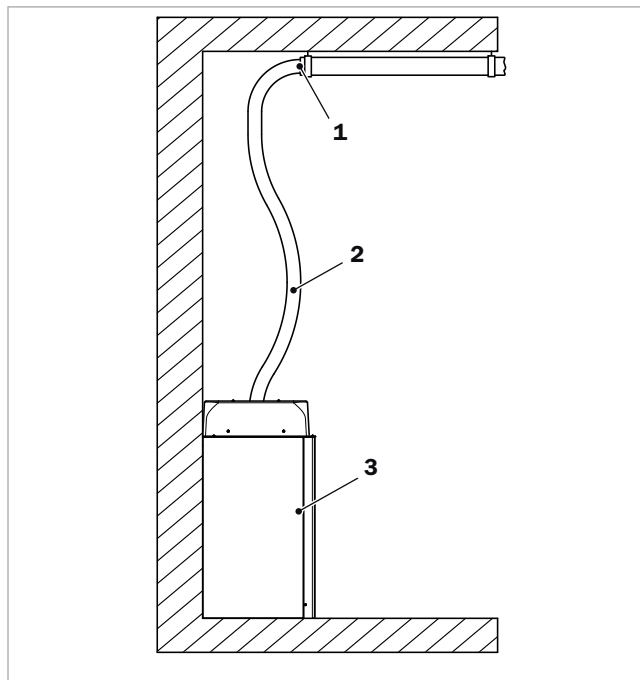
Abb. 56: Schlauchbefestigung Decke mit HT-Rohr
