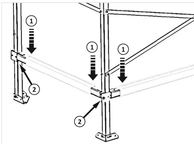
Abb. 80: Gewebe spannen
