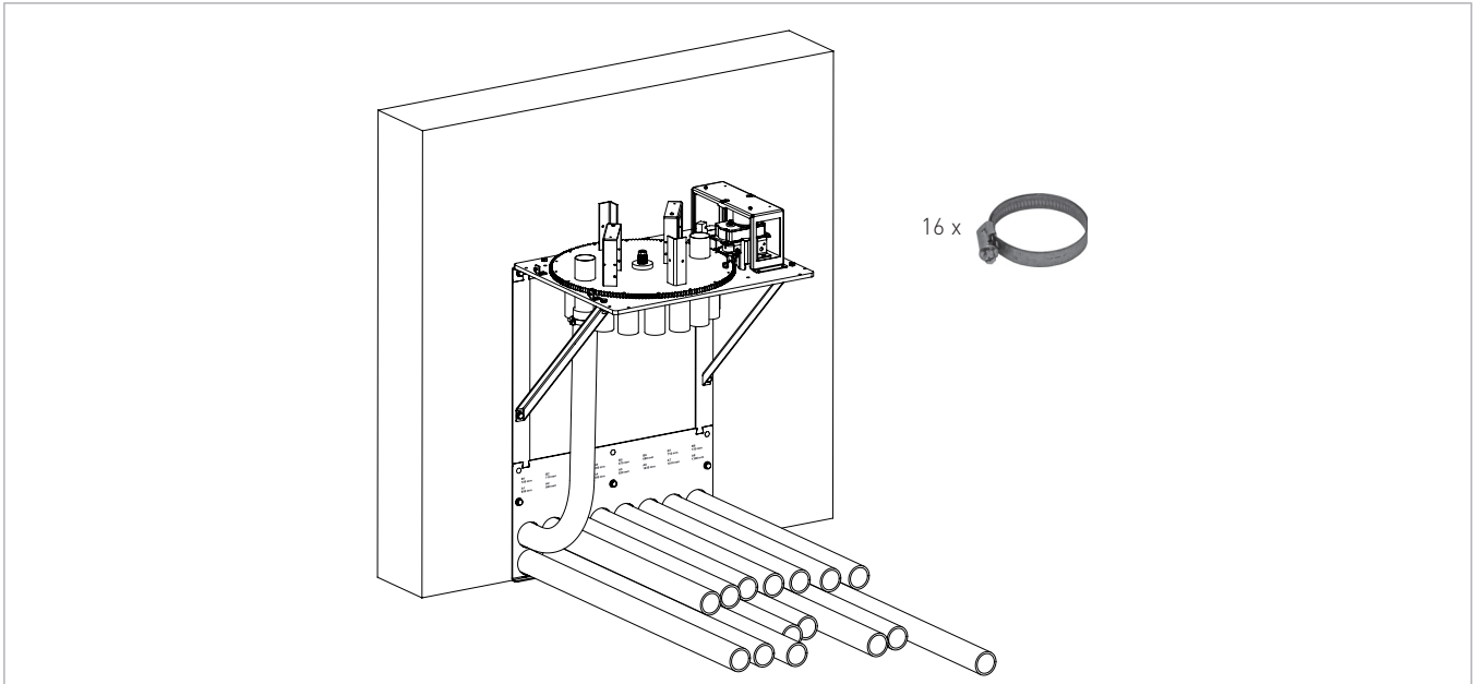
Abb. 51: Schläuche der Reihe nach von B1 bis B8 auf Umschalteneinheit montieren
