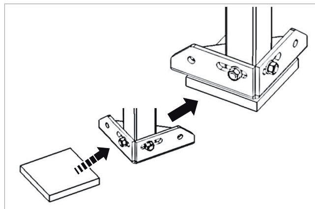
Abb. 81: Dämmplatte unterlegen
