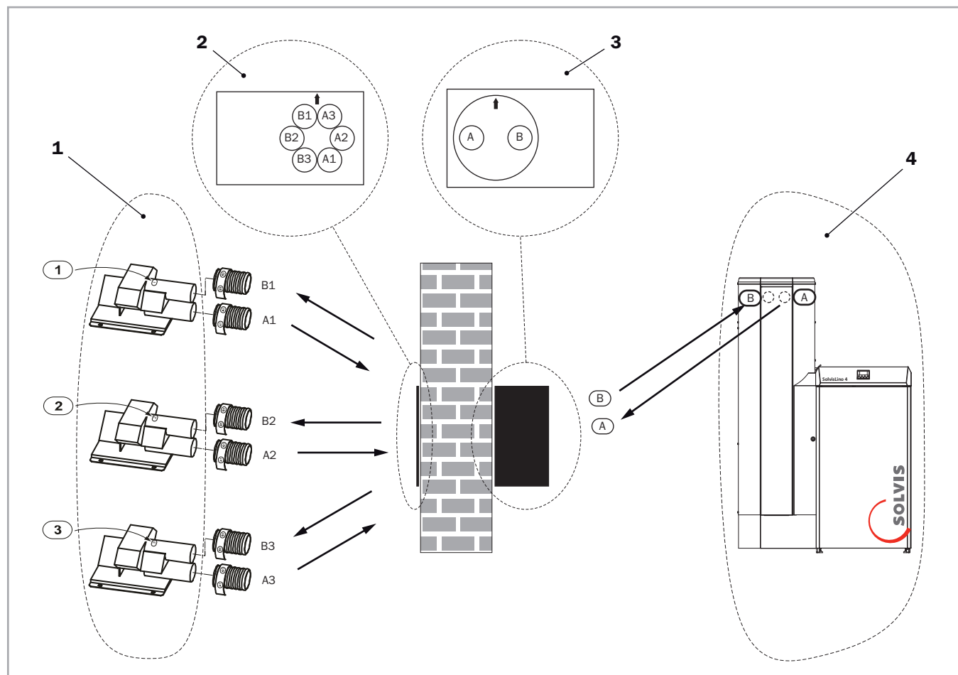
Abb. 6: Anschluss-Übersichtsskizze
