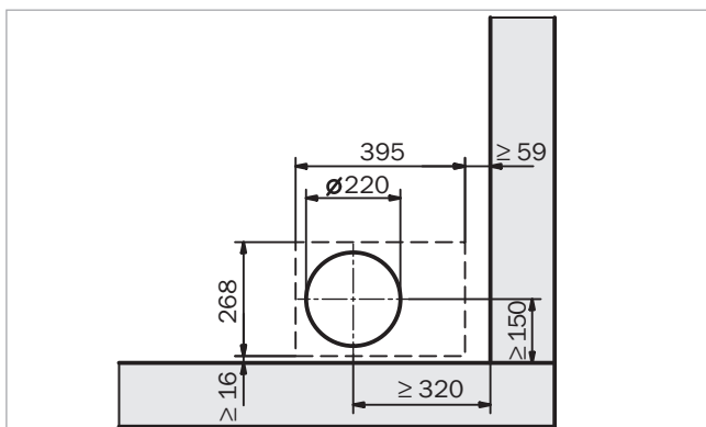
Abb. 12: Mauerdurchführung für Umschalteinheit, Wand rechts – Vorderansicht
