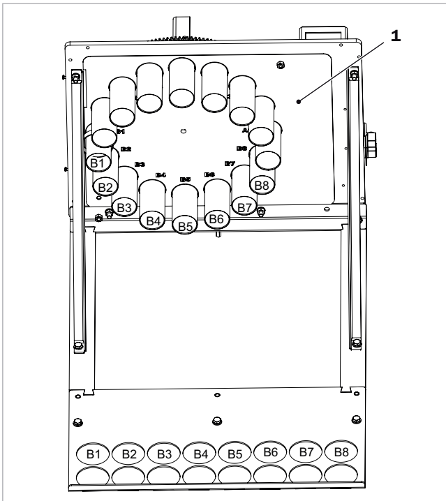
Abb. 52: Rückluftschläuche B1 bis B8 auf Umschalteneinheit montieren - Ansicht von unten
