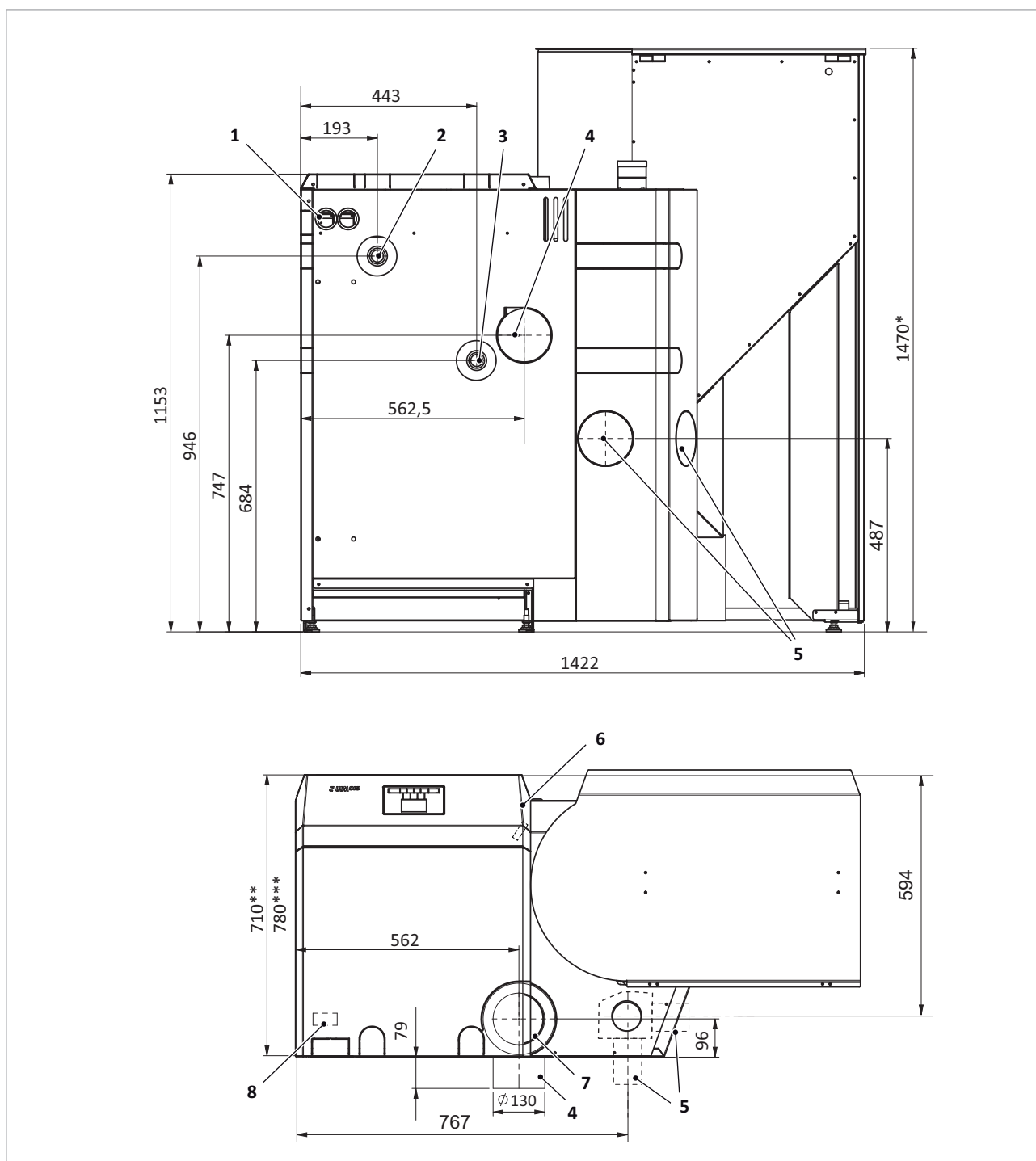
Abb. 21: Ansichten SolvisLino 4 mit Vorratsbeälter (LI-4-xx-VO)
