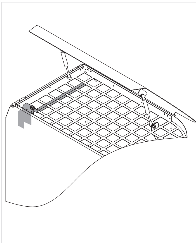
Abb. 15: Schalter montieren
