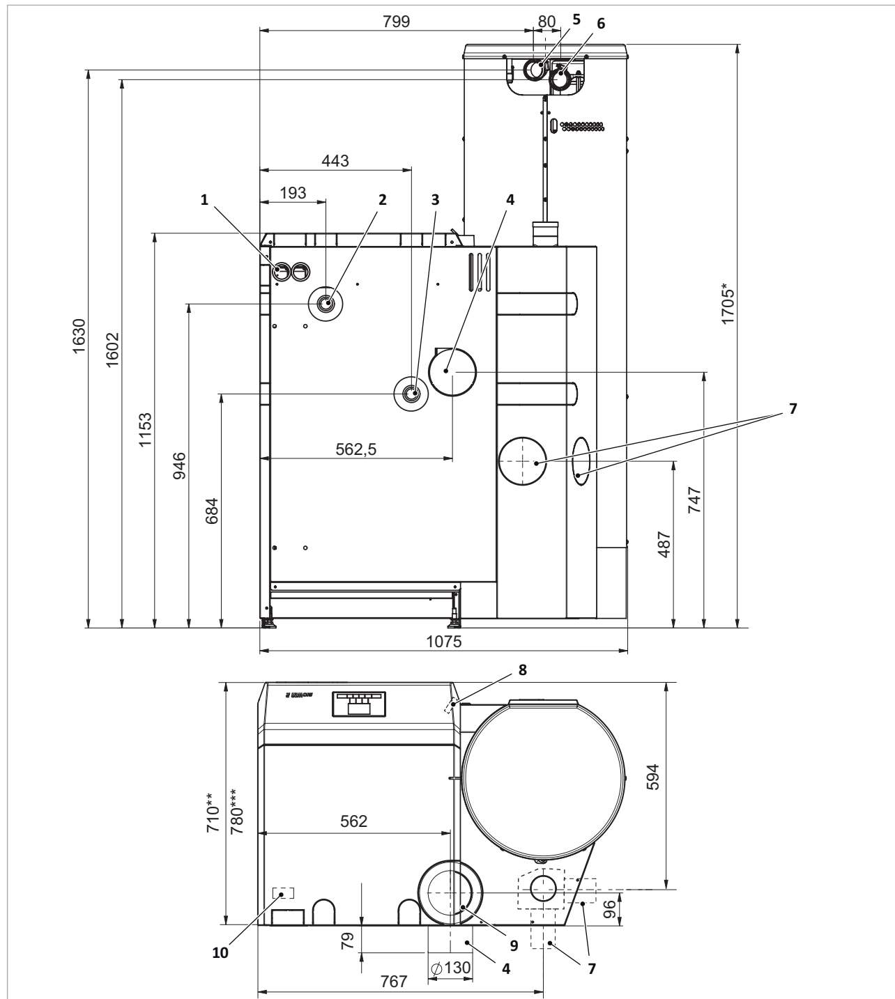
Abb. 20: Ansichten SolvisLino 4 mit Saugturbine (LI-4-xx-GS)
