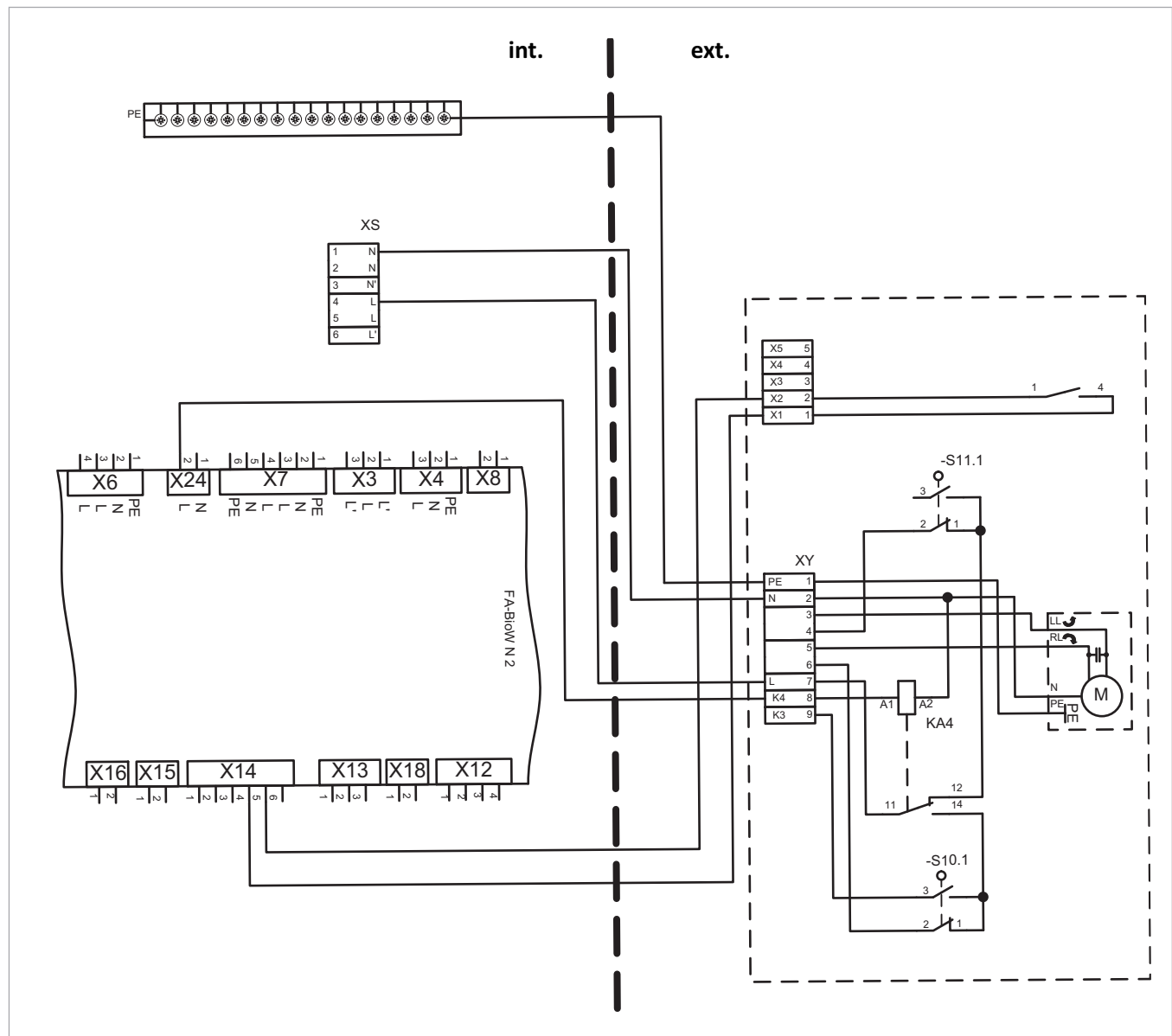
Abb. 18: Anschlussplan Absperreinheit
