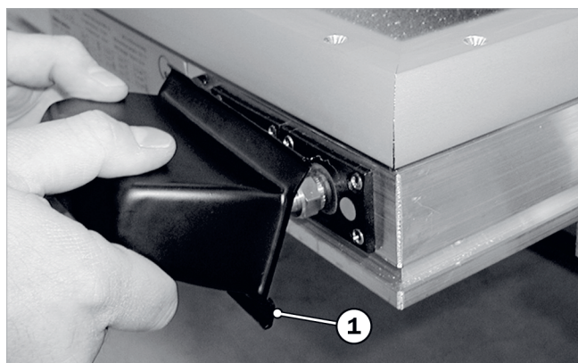
Abb. 51: Abdeckhaube aufsetzen
