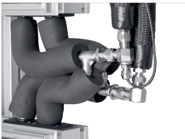
Abb. 53: Über Kreuz installierte Parallelverschraubung
