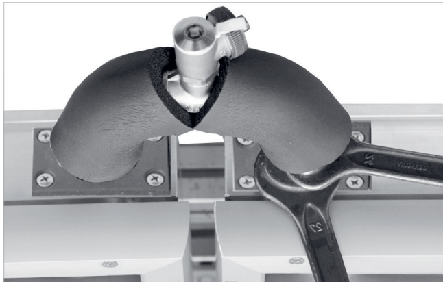
Abb. 67: Verbindung Kollektoren nebeneinander
