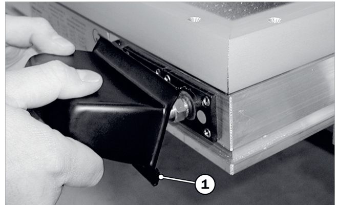
Abb. 46: Abdeckhaube aufsetzen
