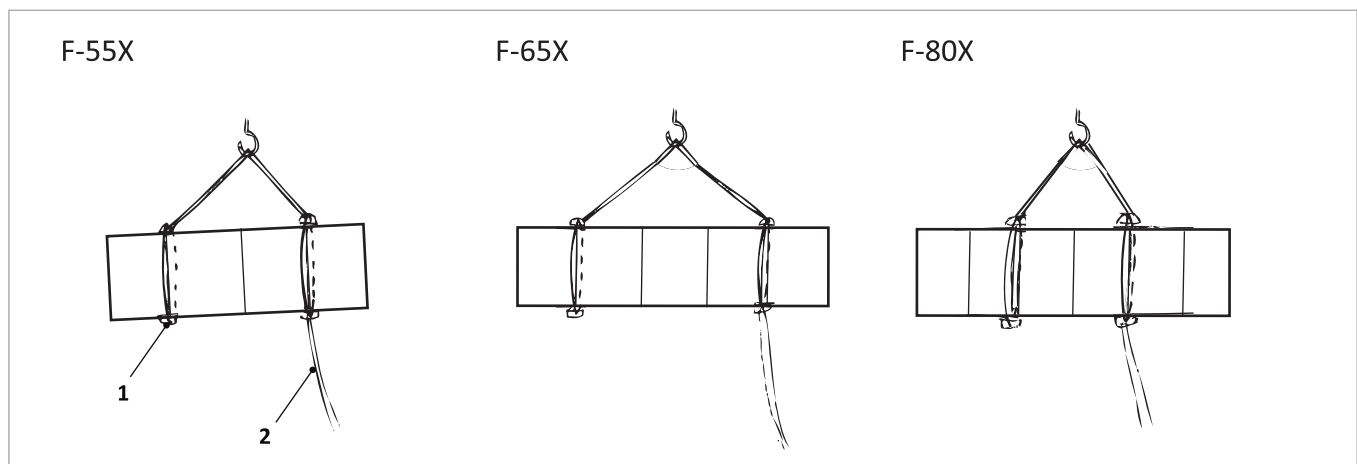
Abb. 2: SolvisFera – Position der Haltegriffe und Schlupfe
