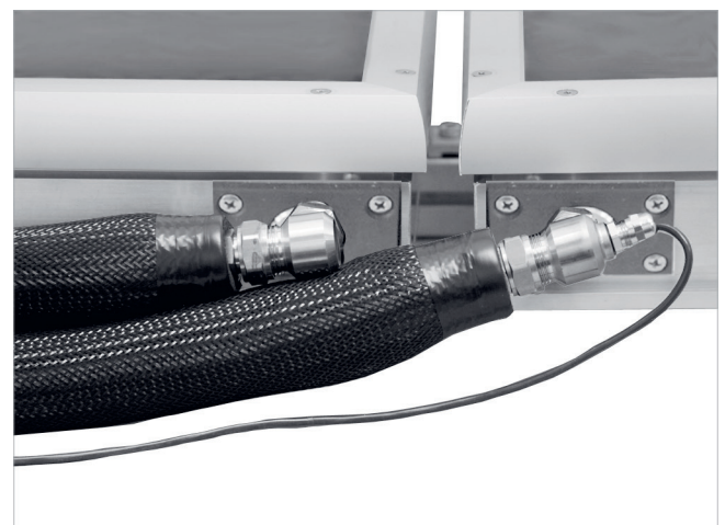
Abb. 66: Flexibler Anschlussrohrsatz mit Isolierung
