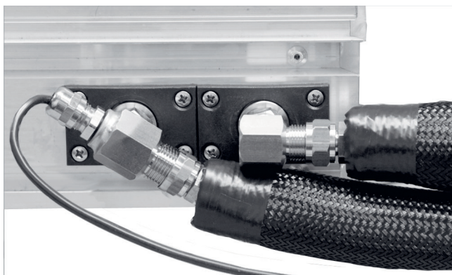
Abb. 44: Flexibler Anschluss mit Isolierung
