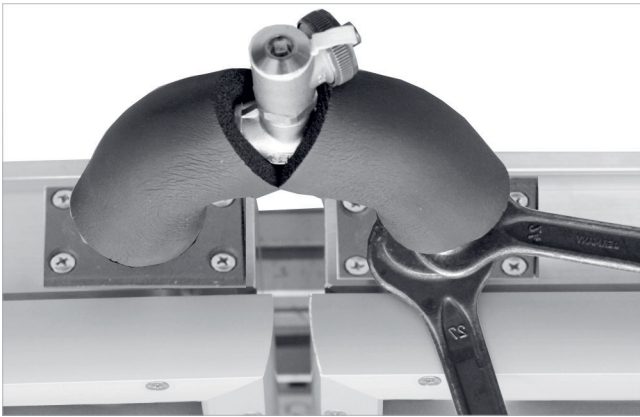
Abb. 64: Verbindung Kollektoren nebeneinander
