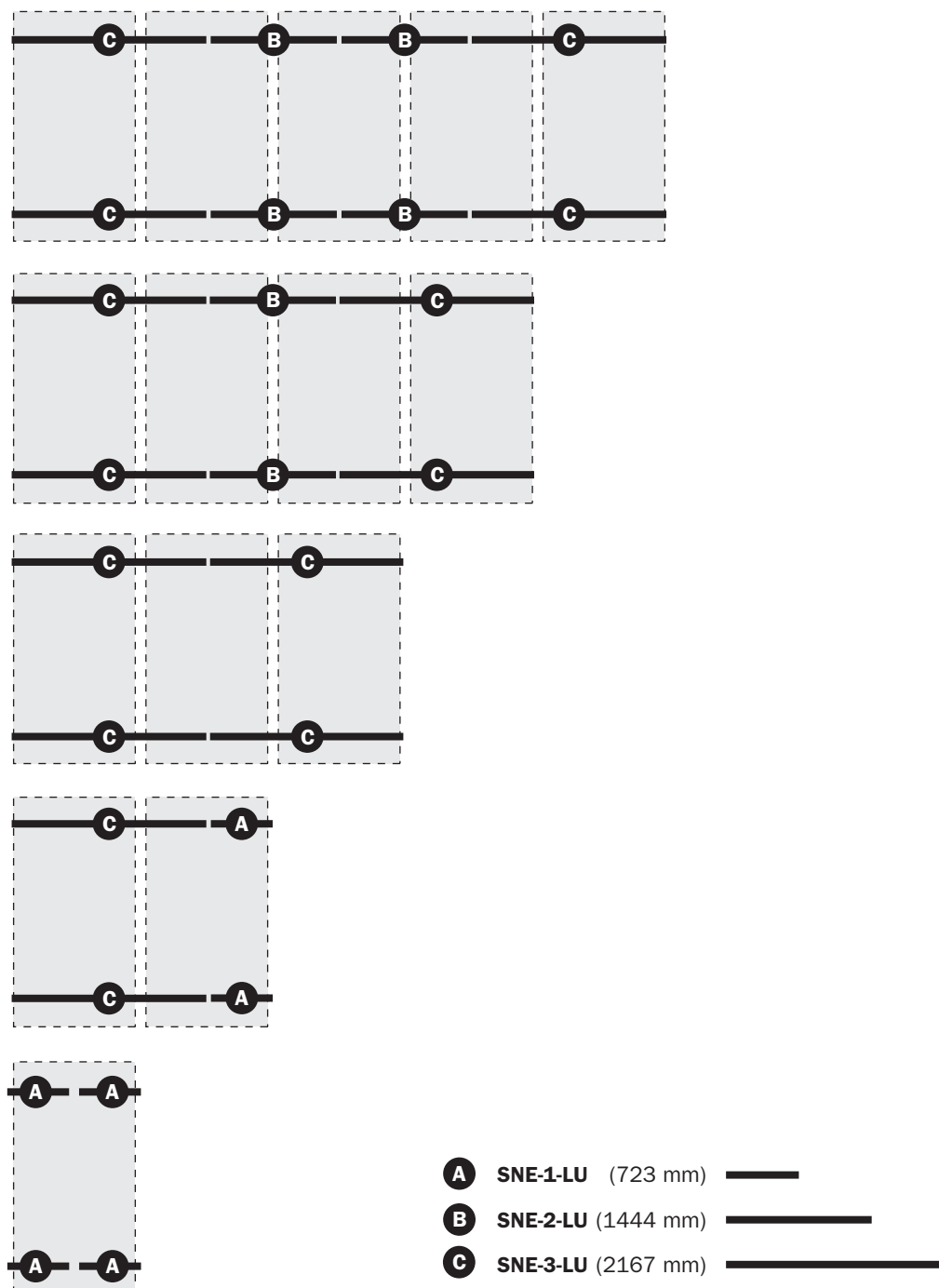
Abb. 13: Kombination der Halteschienenpaare für SolvisLuna
