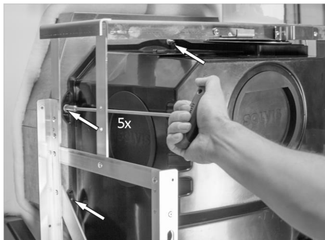
Fig. 25: Serraggio della copertura della camera di aspirazione
