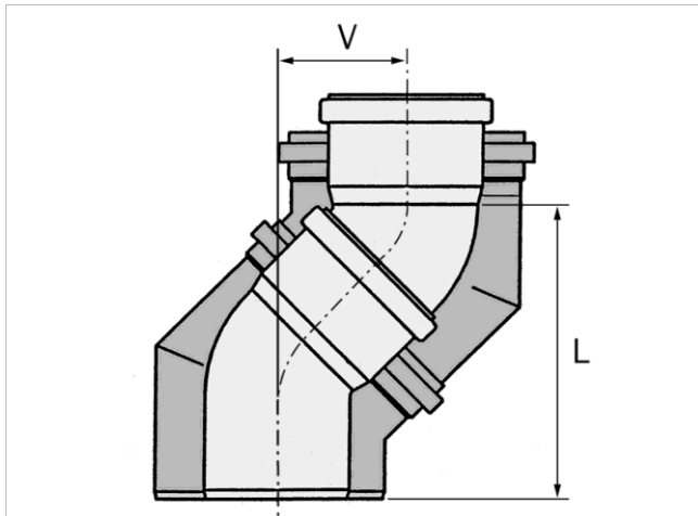
Fig. 29: Spostamento e lunghezza
