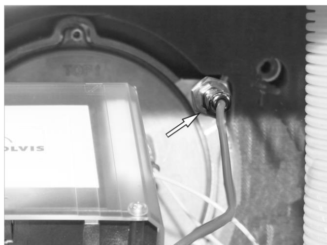
Fig. 34: inserimento dell'eSTB
