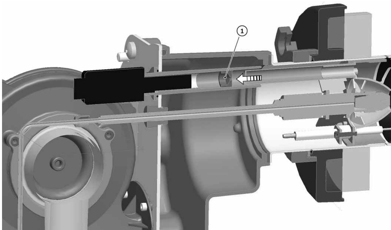
Abb. 1: Schnitt durch den Brenner / Section through the burner/ Sezione attraverso il bruciatore/ Sección a través del quemador / Seção através do queimador / Section à travers le brûleur / Doordnede door de brander
