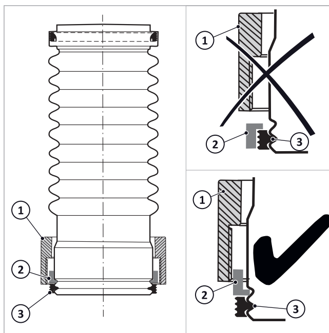
Afb. 17: Schroefkoppeling opgestoken
