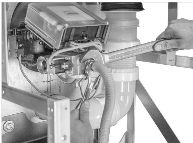
Afb. 23: Gasleiding aansluiten
