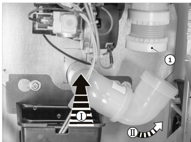
Afb. 18: De rookgasbocht monteren
